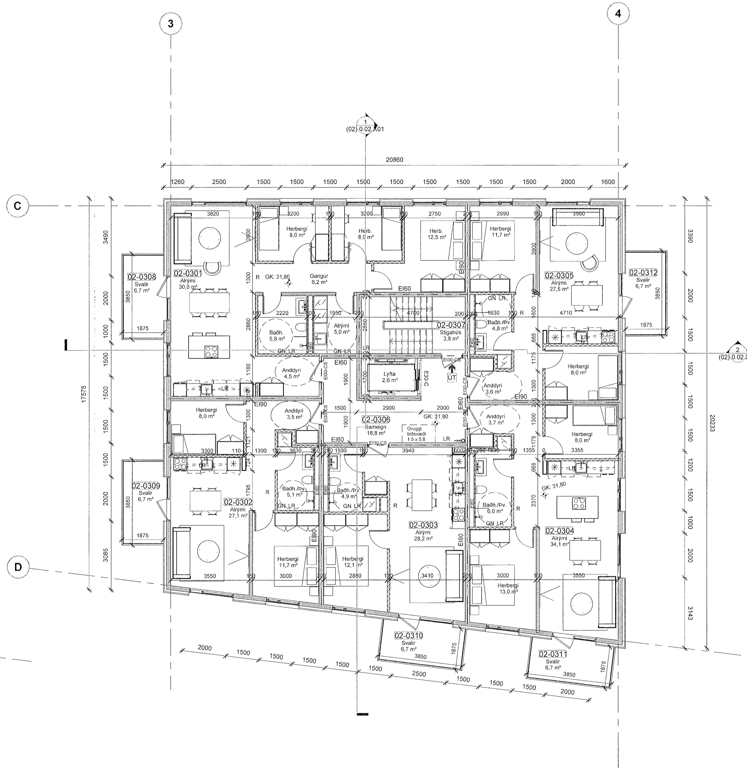
03-Hæð 3 - mhl 2 1 : 100
