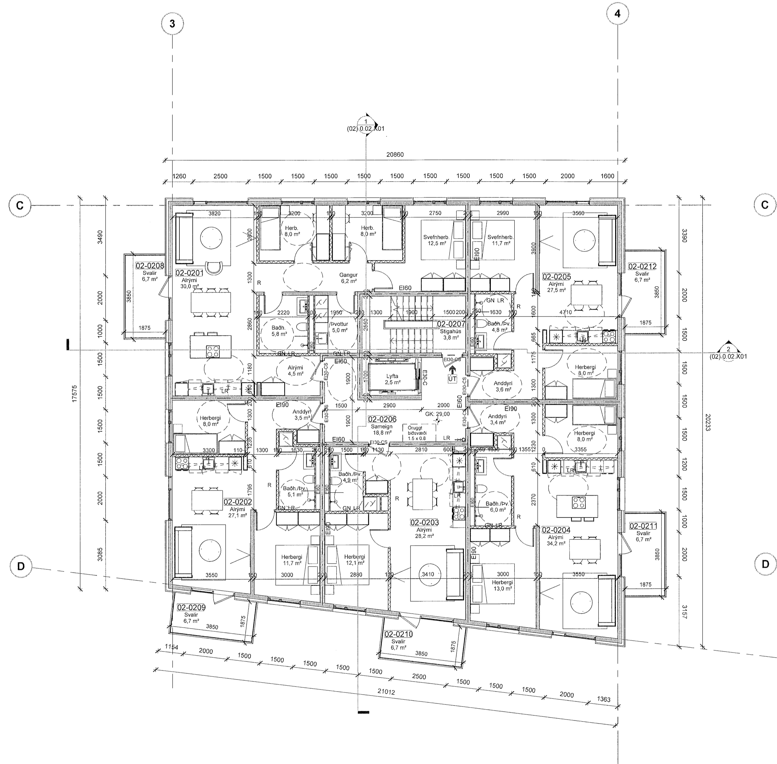
02-Hæð 2 - mhl 2 1 : 100
