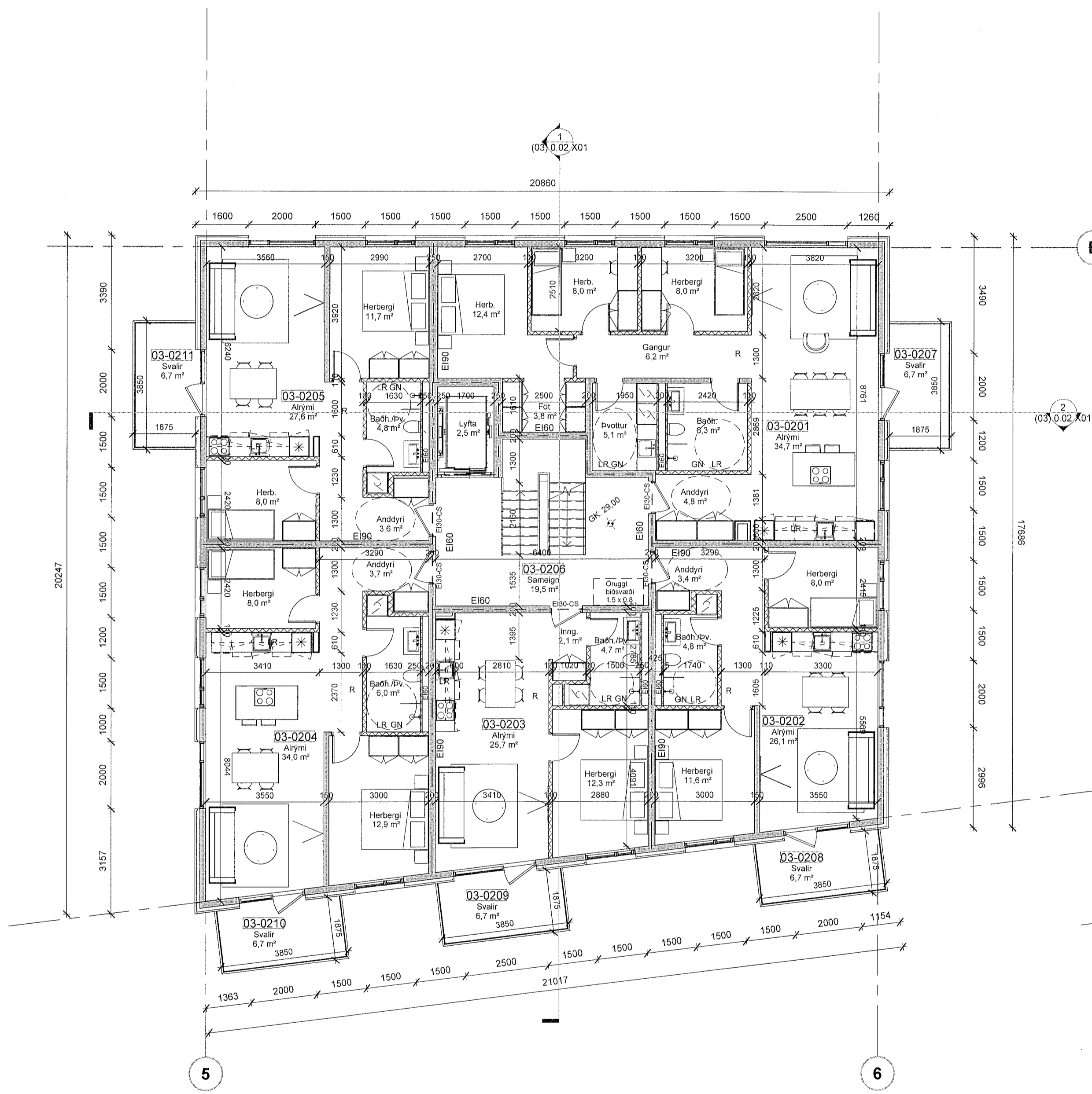
02-Hæð 2 - mhl 3 1:100
