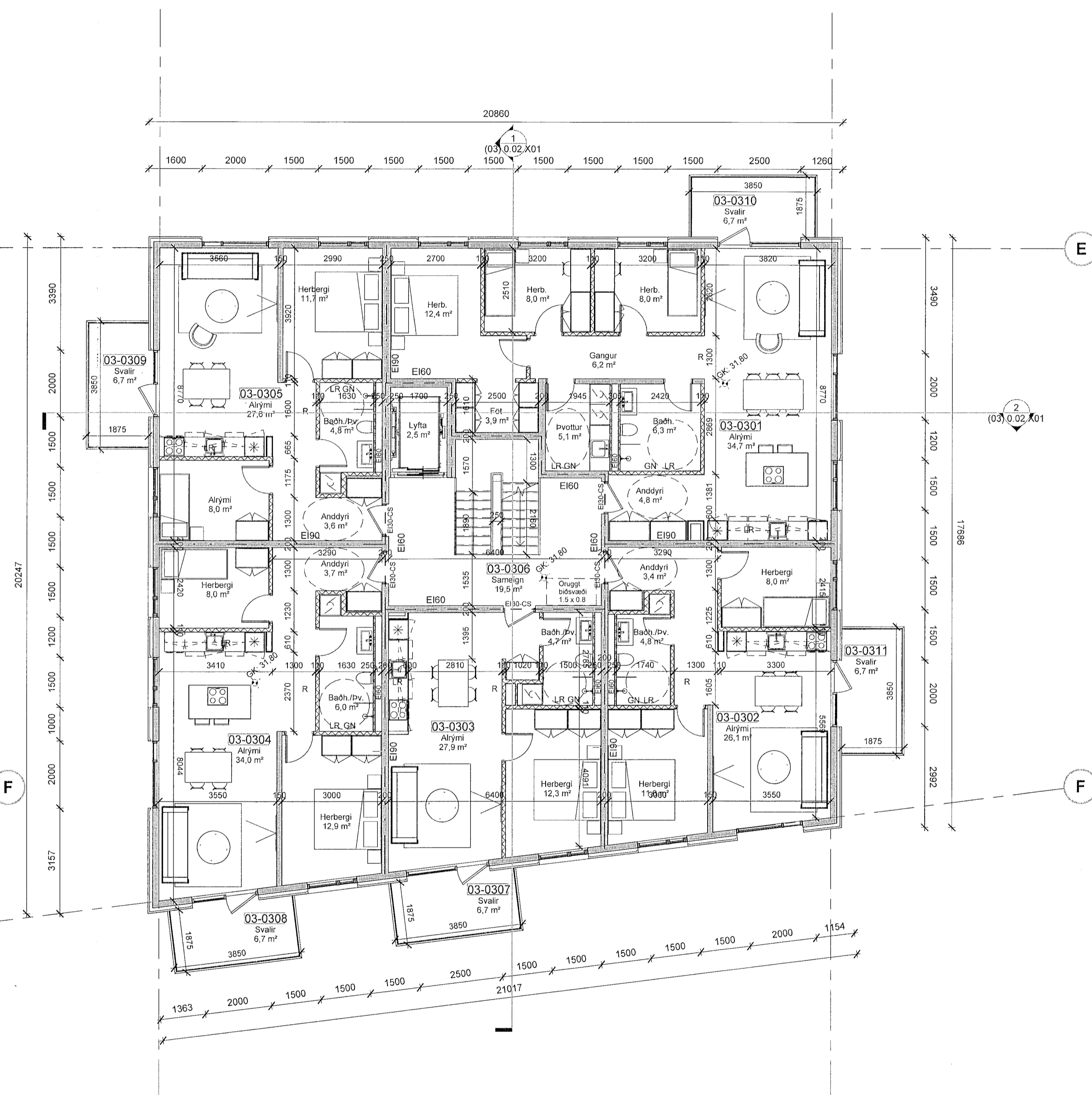
03-Hæð 3 - mhl 3 1:100
