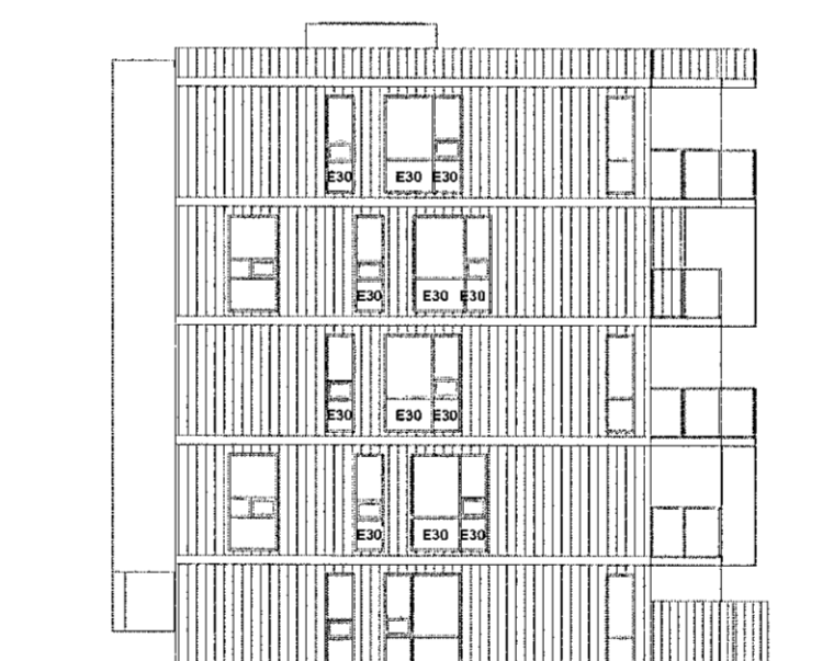
Vestur- 1 : 200
