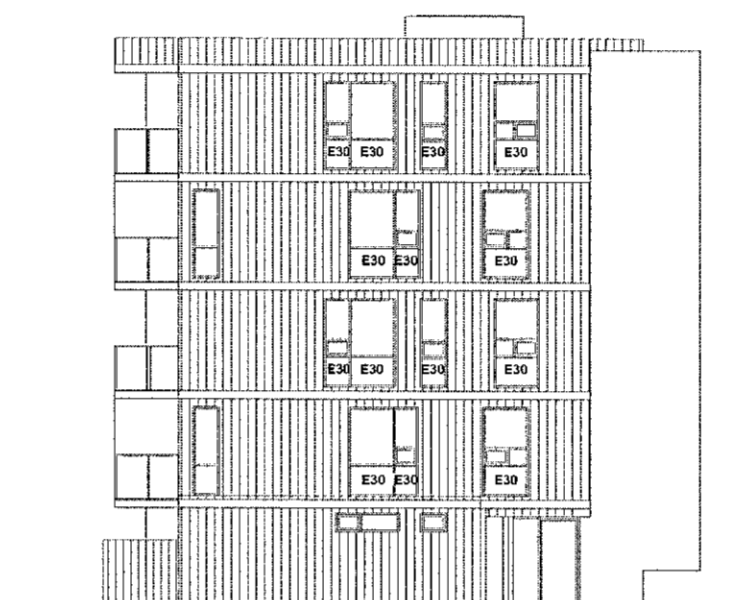
Austur- 1 : 200
