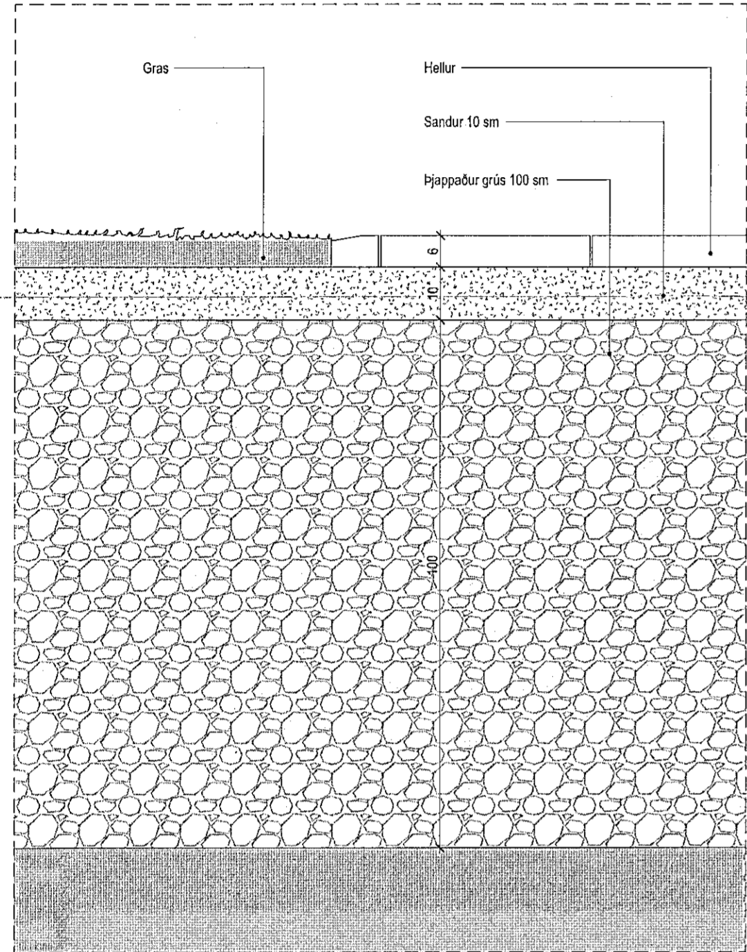
Skýrimynd: uppbygging akumuleiða slökkvibíla 1:10
