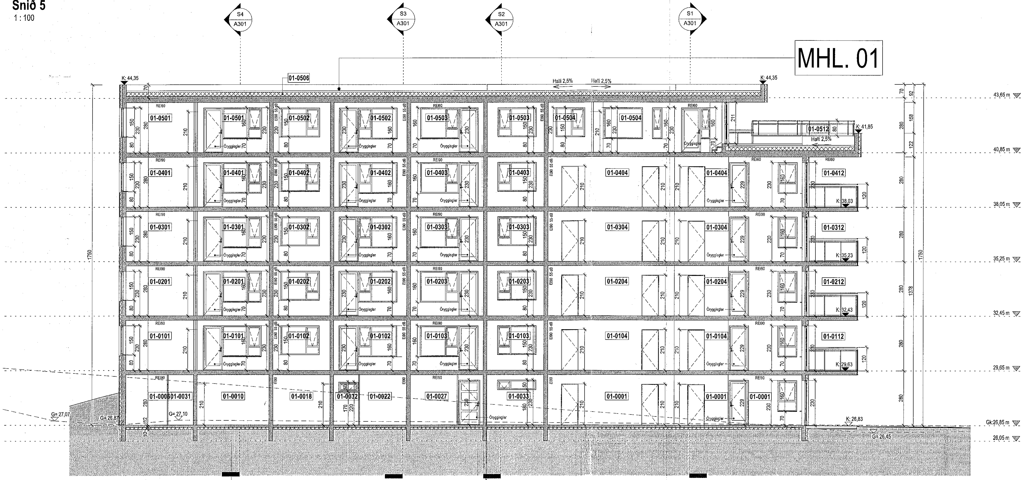
Snið 6 1:100
