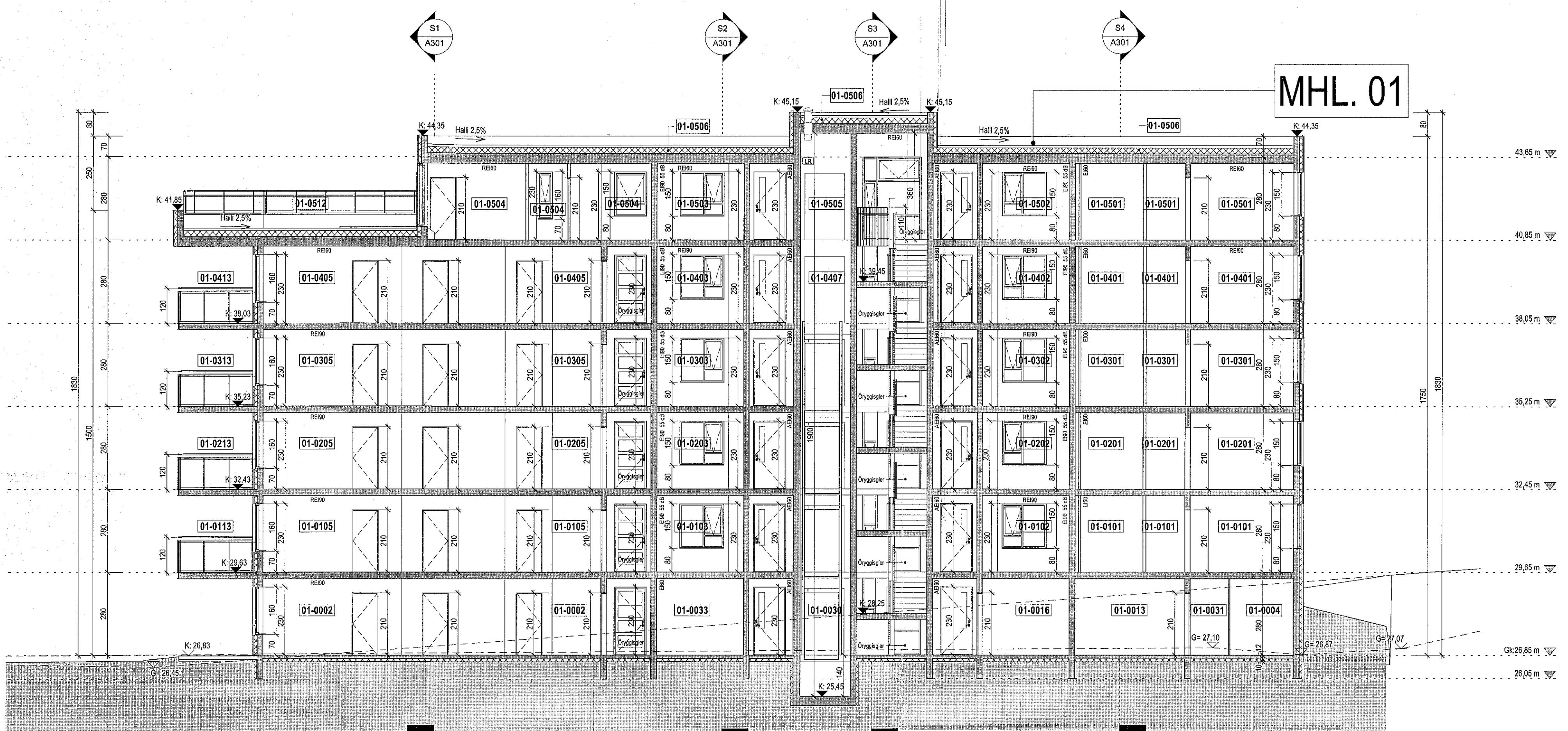
Snið 5 1:100
