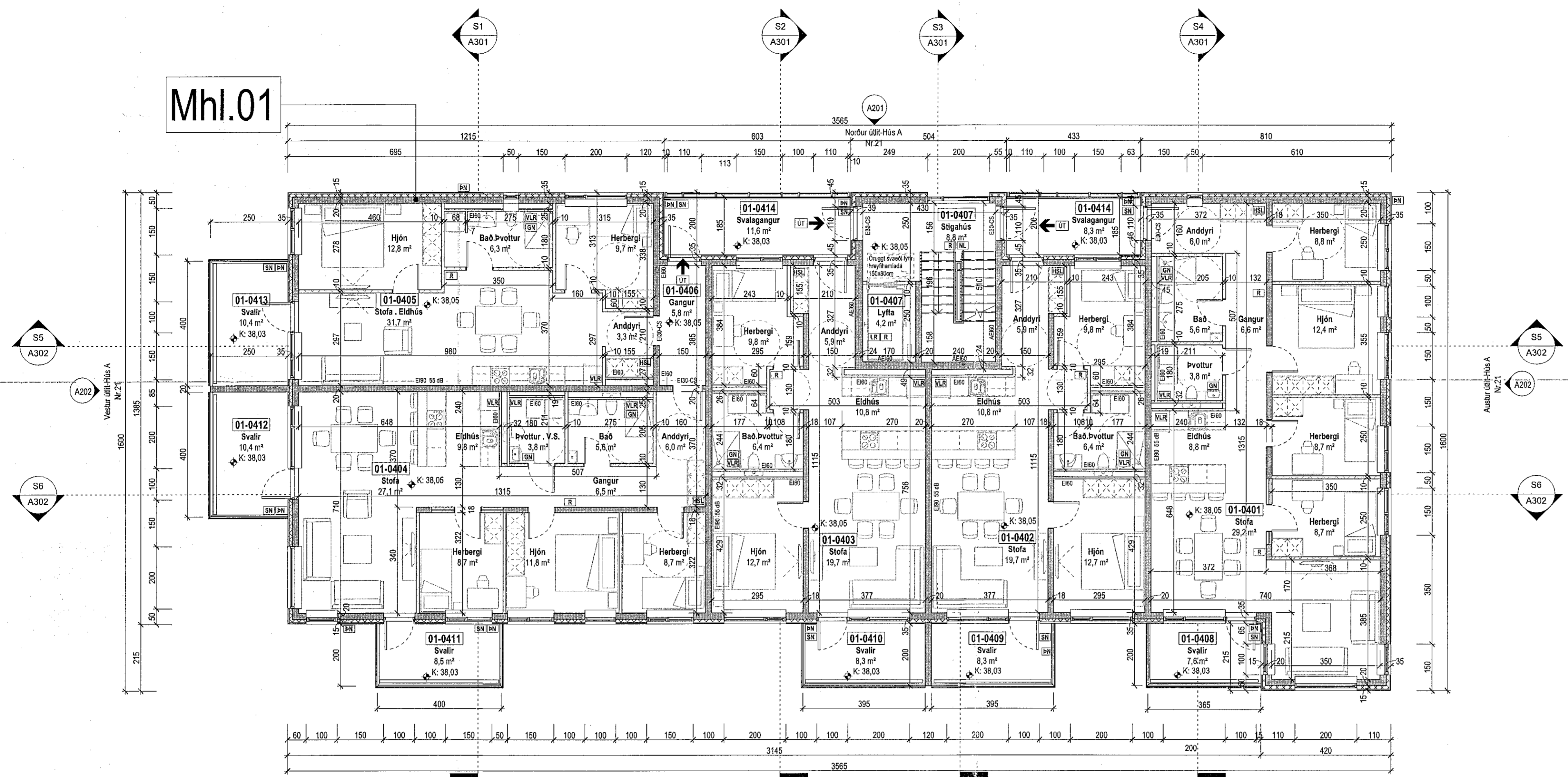
Grunnmynd 4.hæð 1:100
