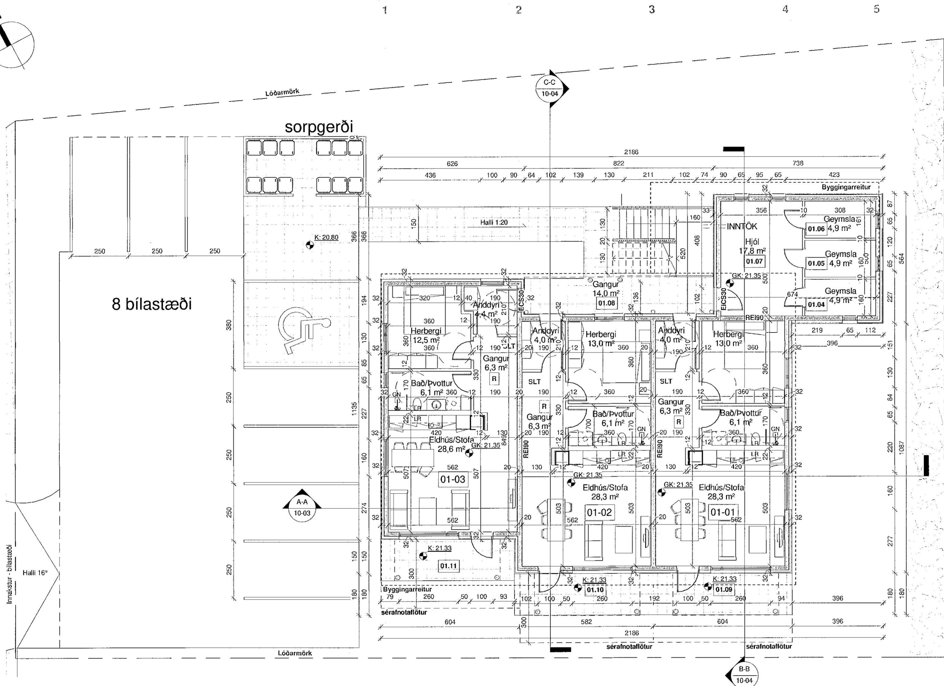
Grunnmynd 1. hæð 1 : 100
