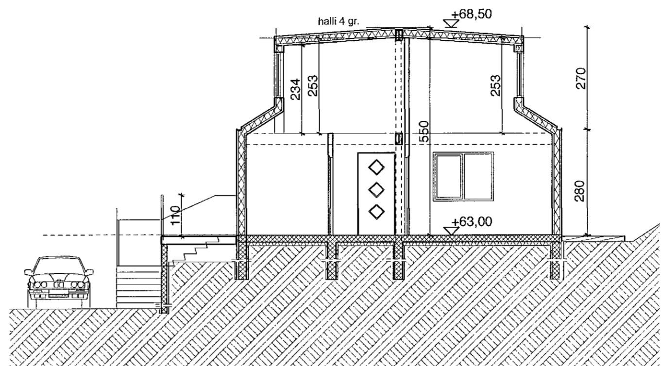
B SNEIDING 1:100
