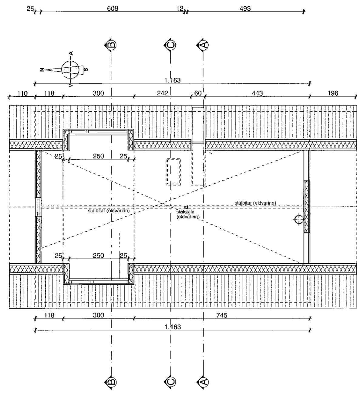
LÁRÉTT SNID Í ÞAK 1:100
