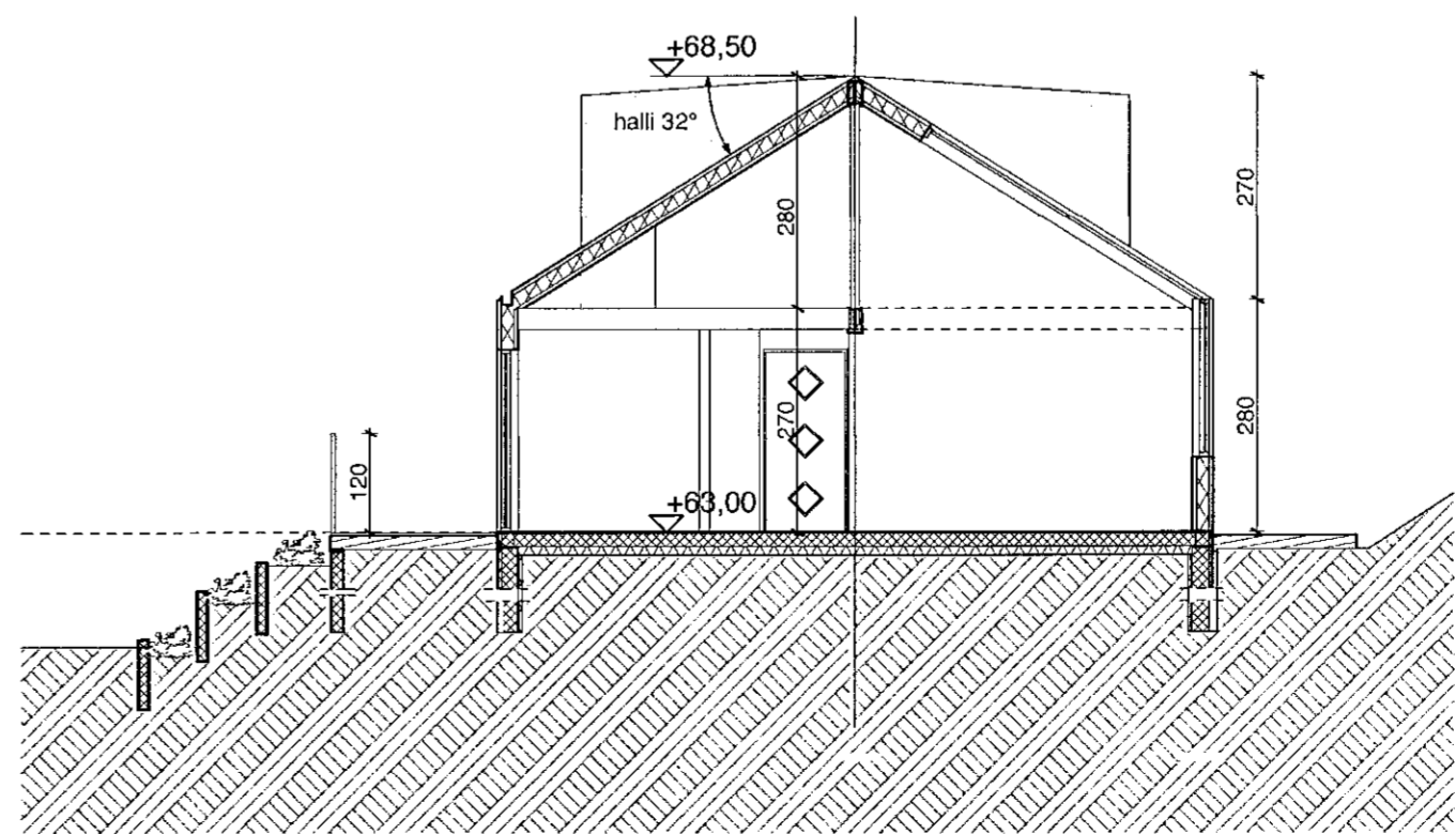
A SNEIDING 1:100
