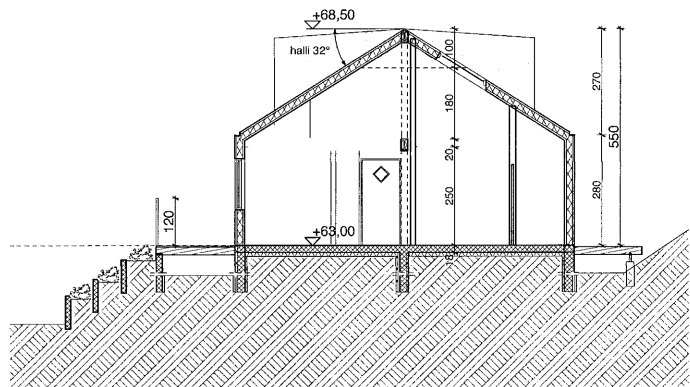
C SNEIDING 1:100
