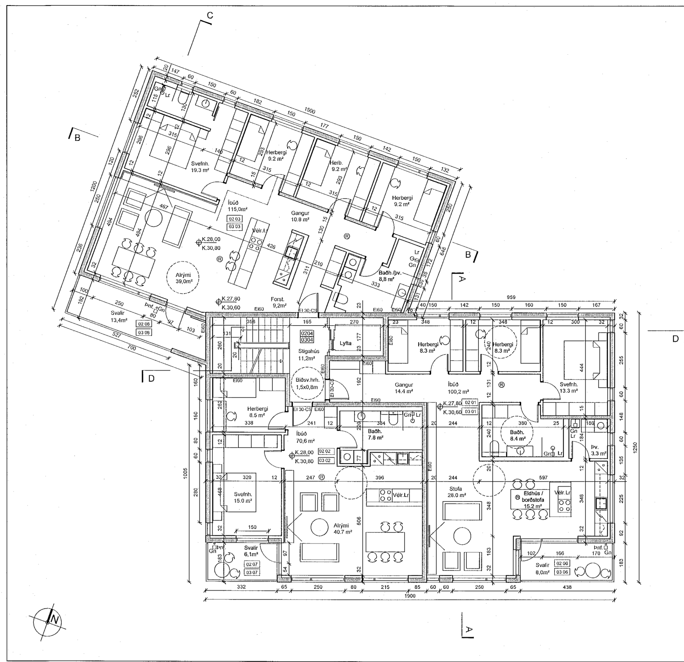
GRUNNMYND 2-3 HÆÐ
