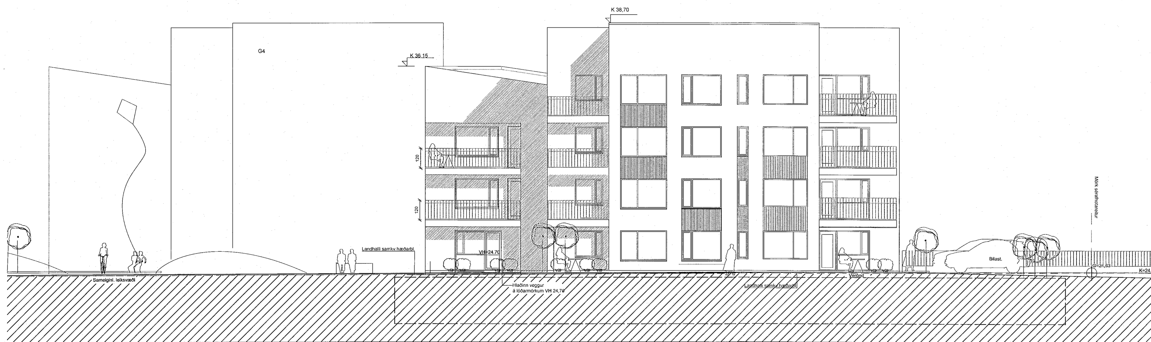
ÚTLIT SUÐUR
