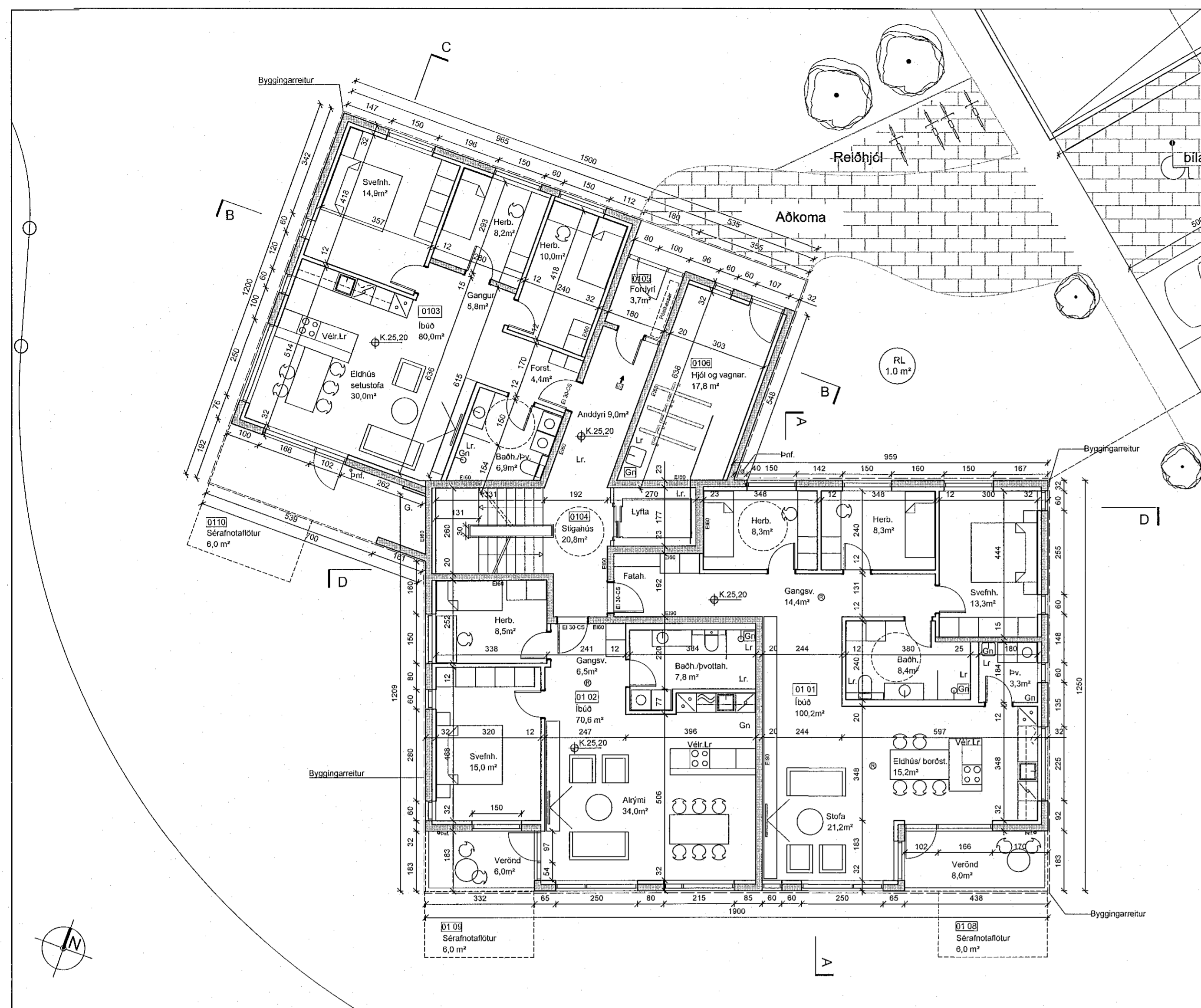
GRUNNMYND 1.HÆÐ
