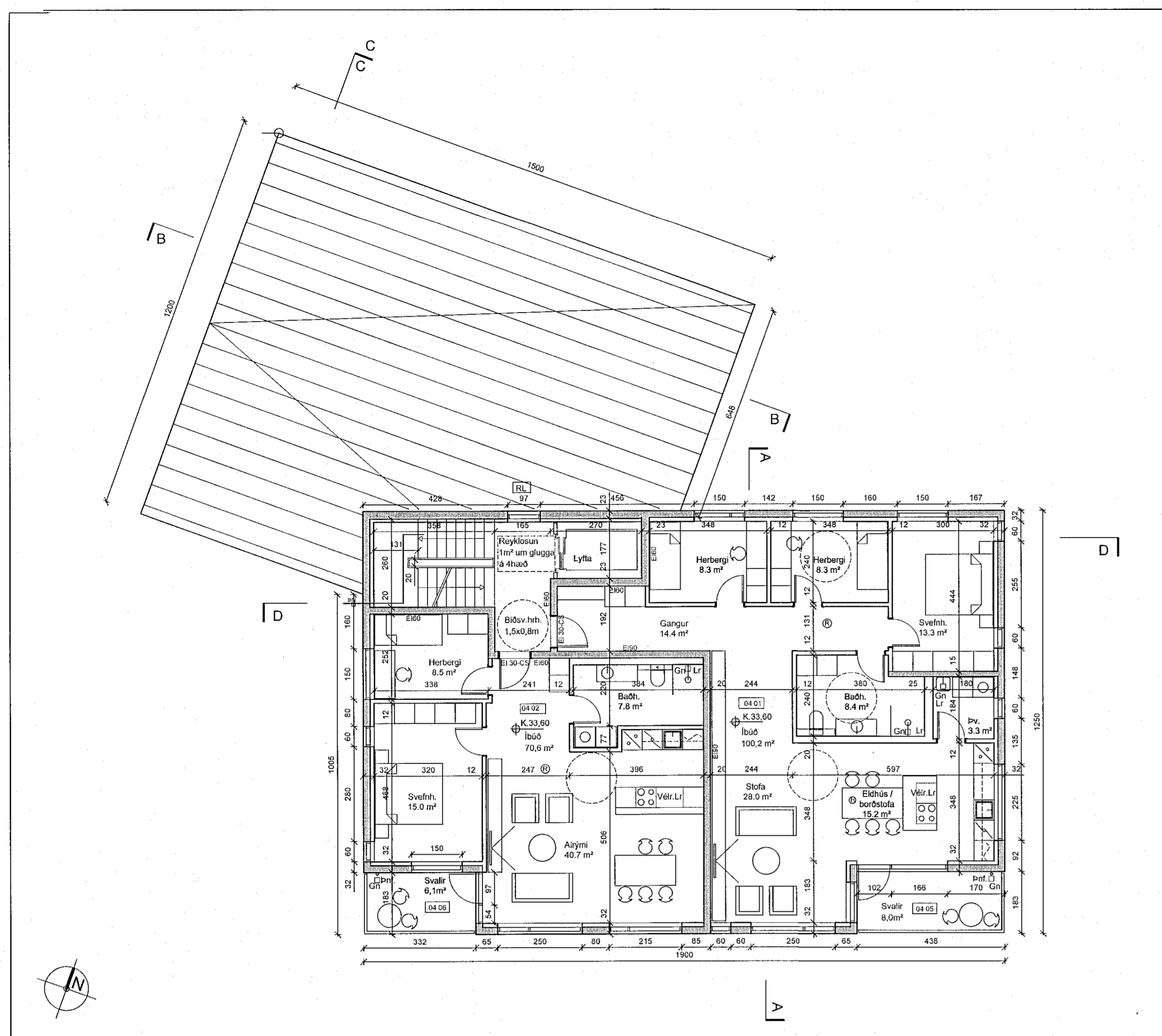
GRUNNMYND 4 HÆÐ
