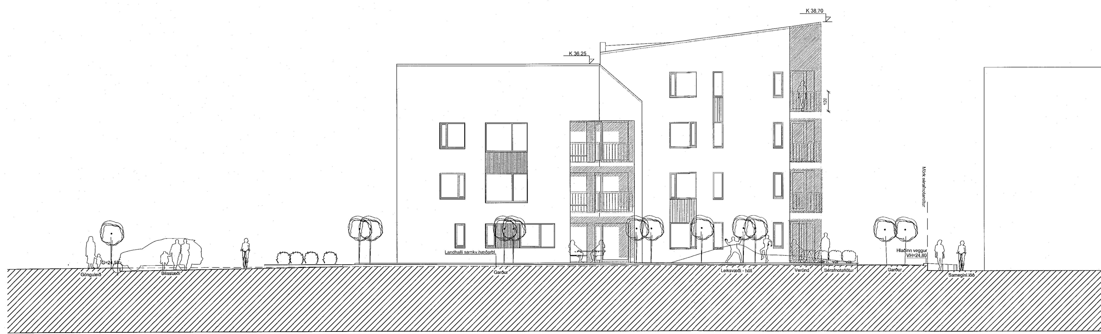
ÚTLIT VESTUR
