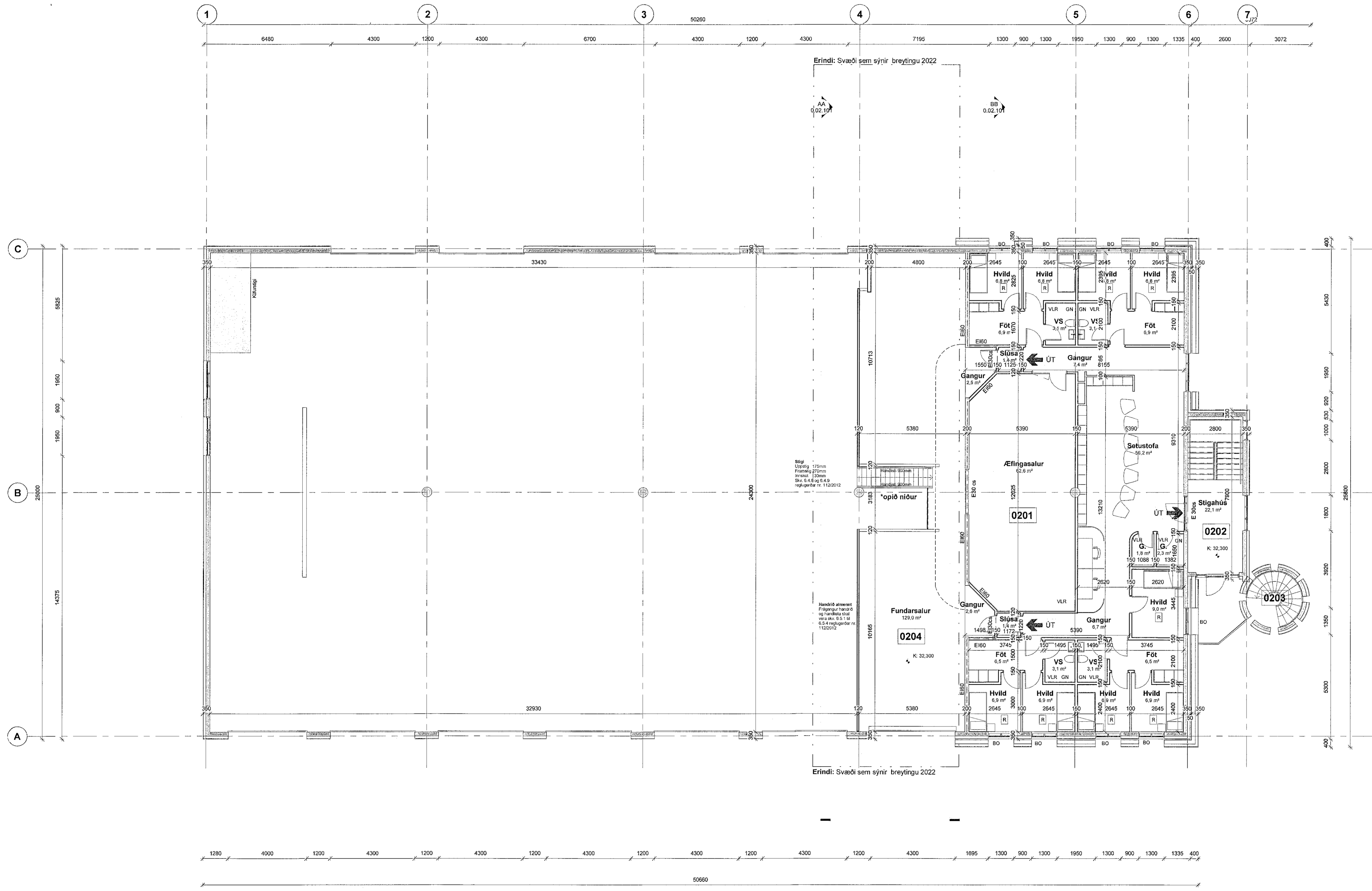
GRUNNMYND 2.HÆÐAR 1:100
