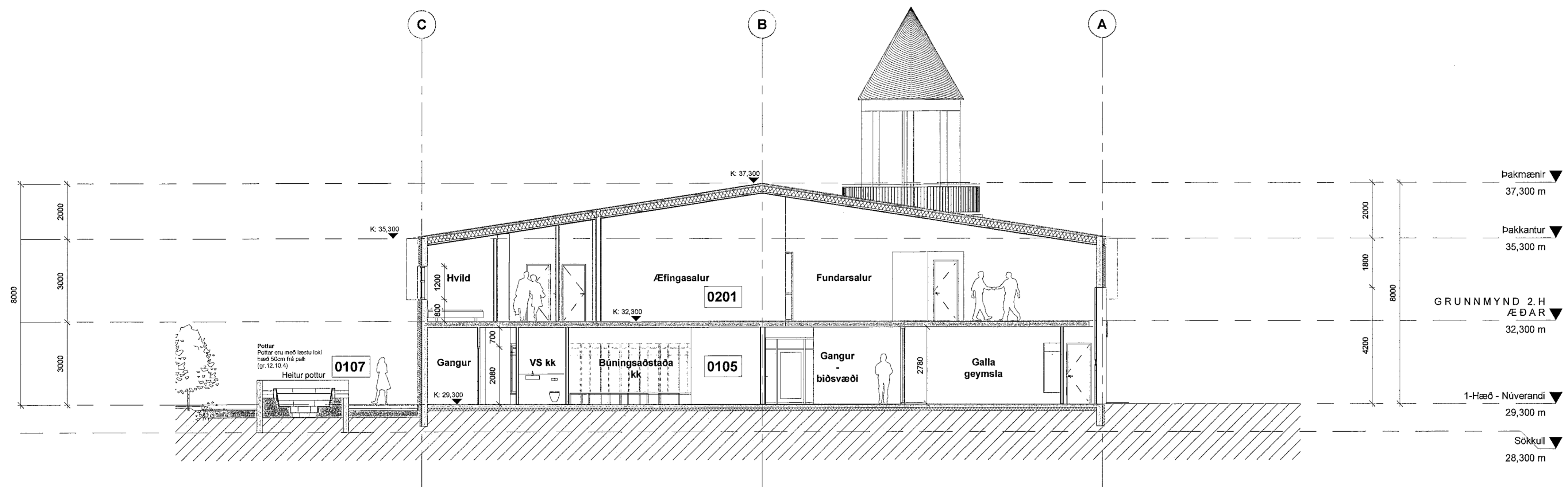
SNEIDING BB 1:100
