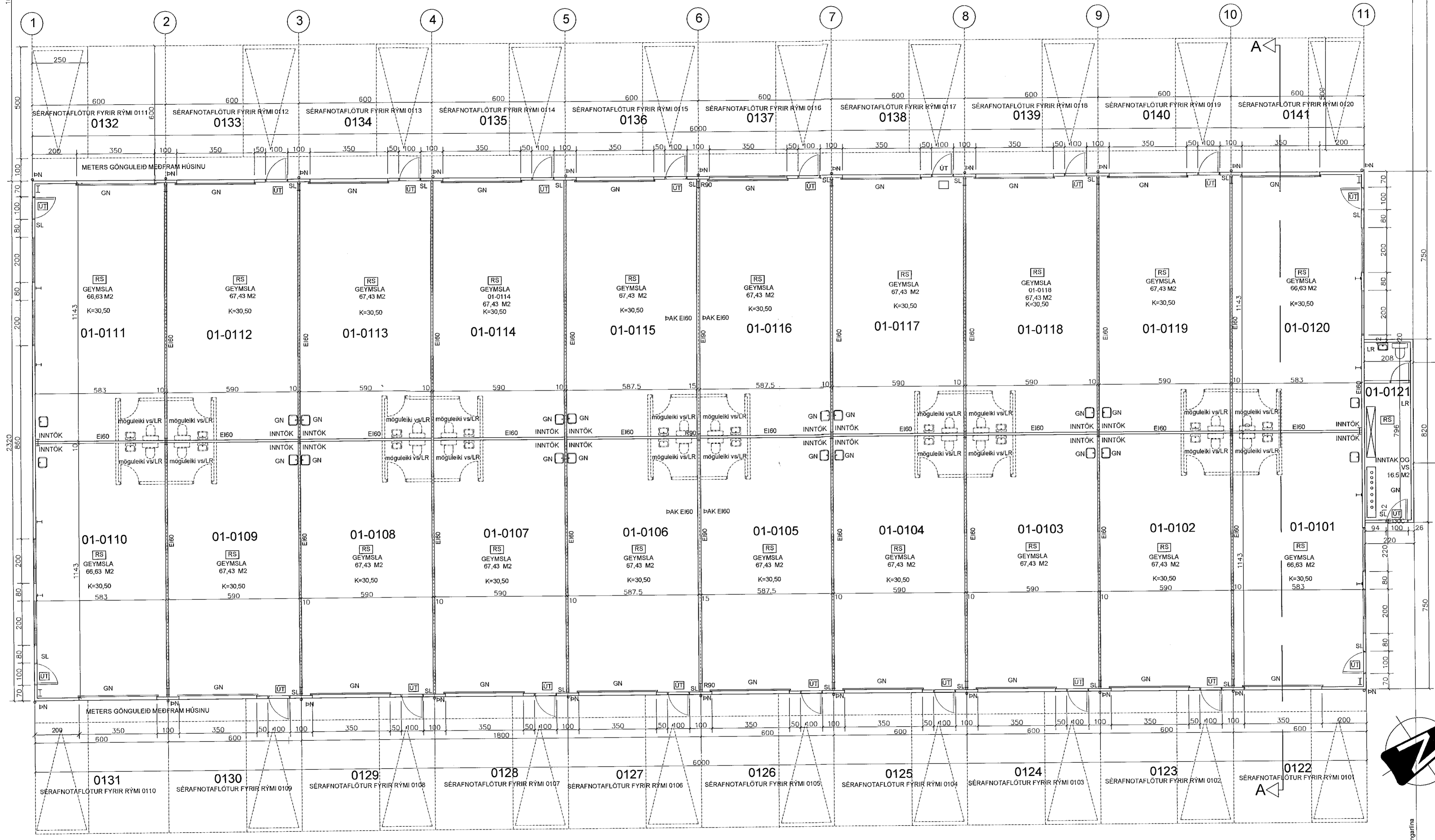
GRUNNMYND 1:100
