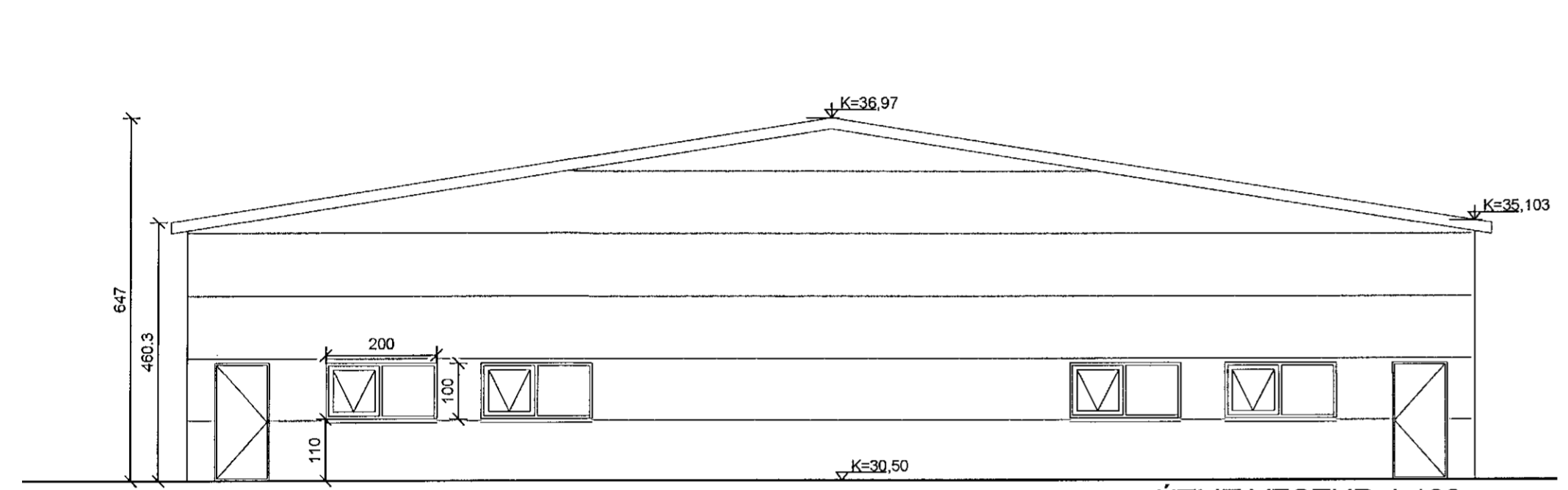
ÚTLIT VESTUR 1:100
