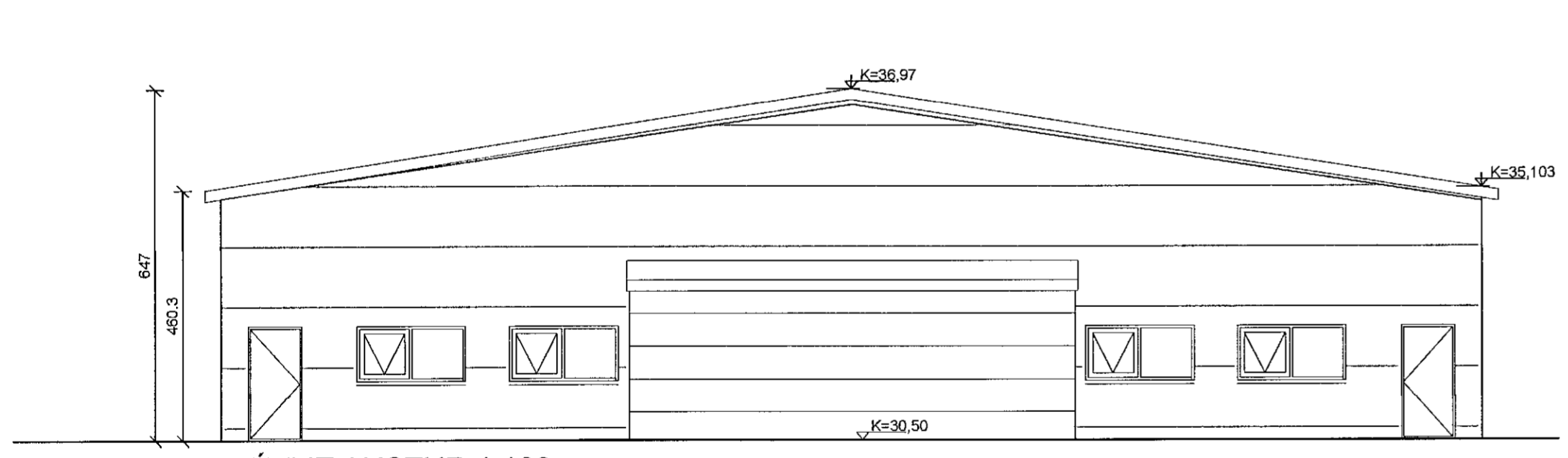
ÚTLIT AUSTUR 1:100
