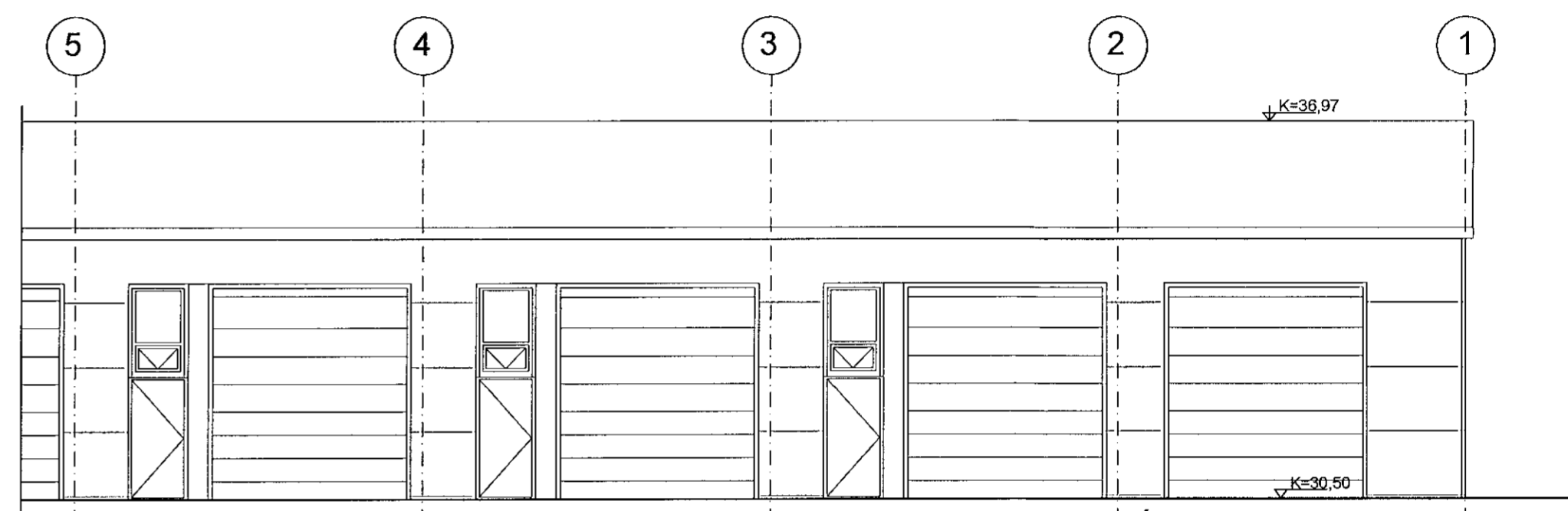
ÚTLIT NORÐUR 1:100
