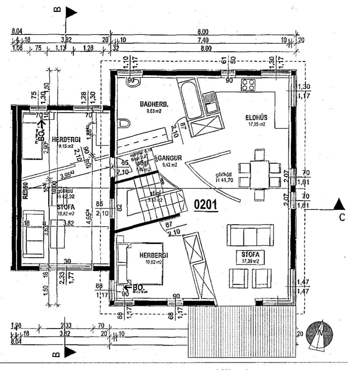
Grunnmynd 2. hæð 1:100
