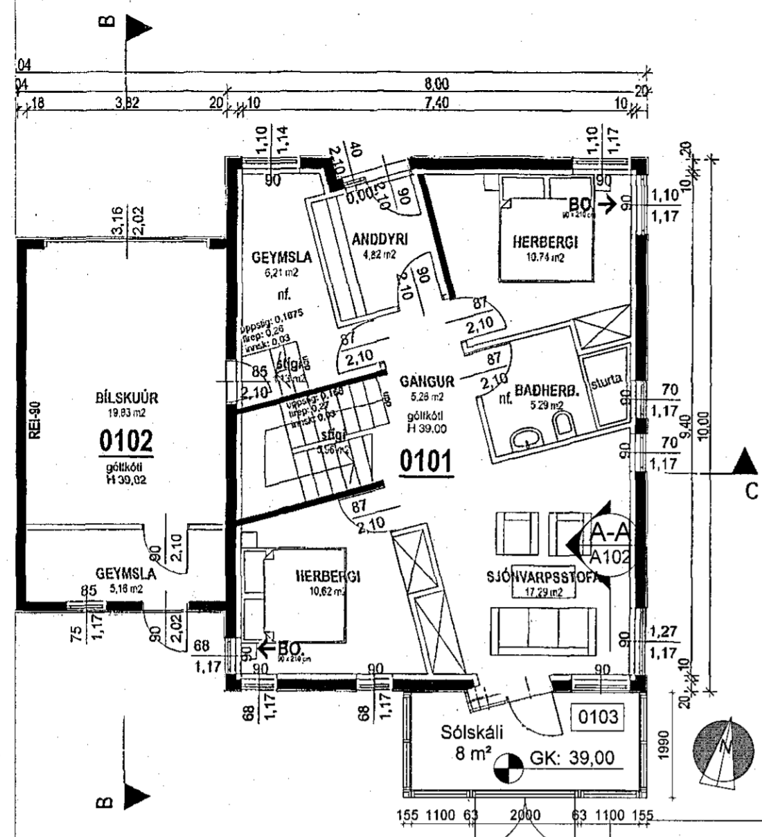
Grunnmynd 1st. hæð 1:100
