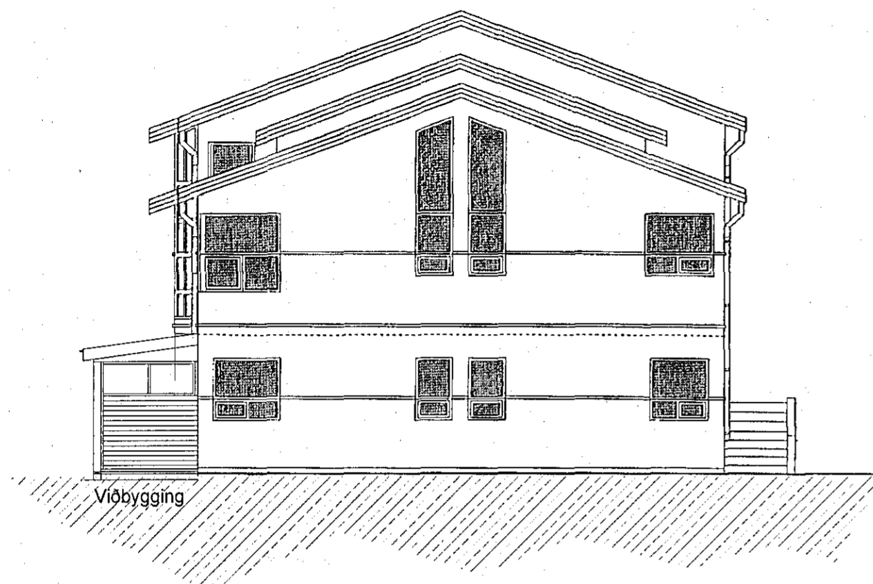
Ásýnd austur 1:100
