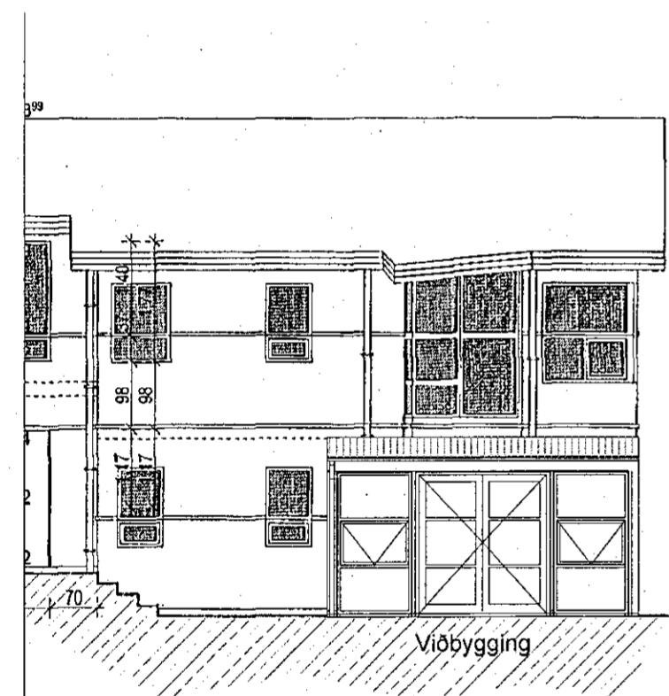
Ásýnd suður 1:100
