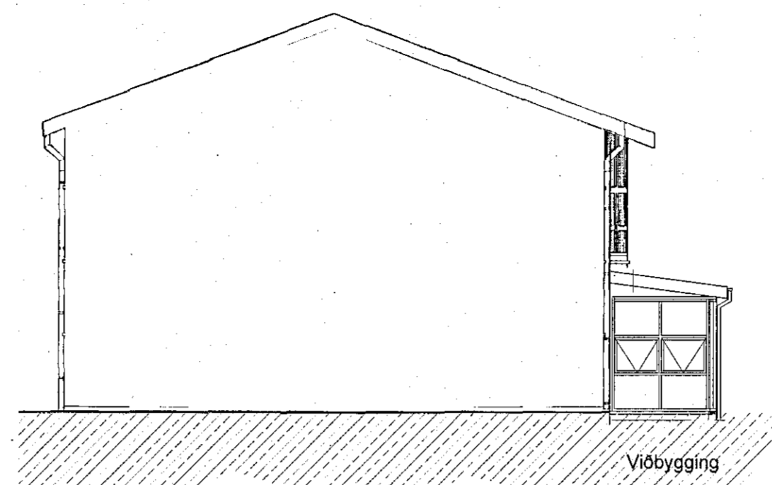
Ásýnd vestur 1:100
