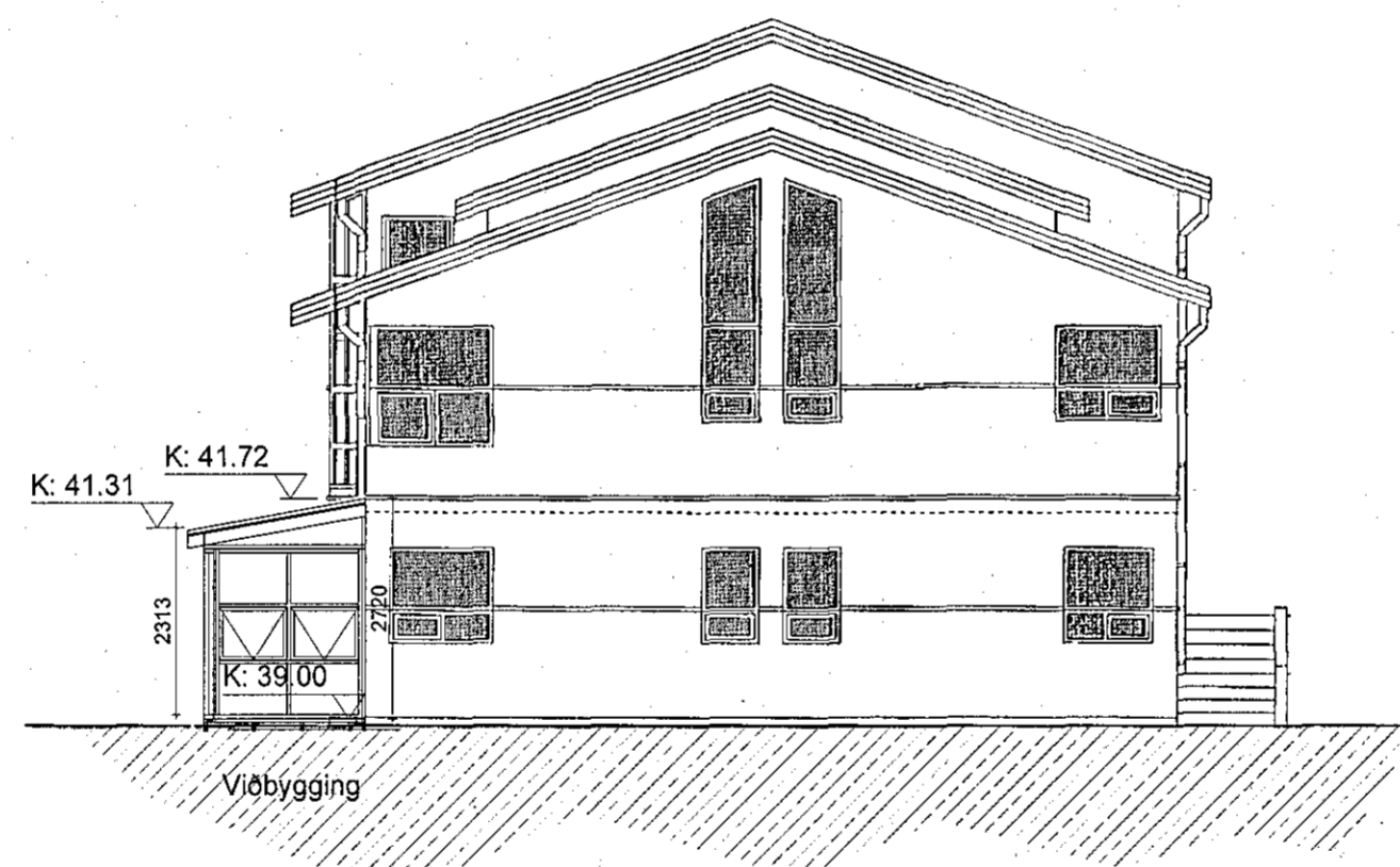
Snið A-A 1:100
