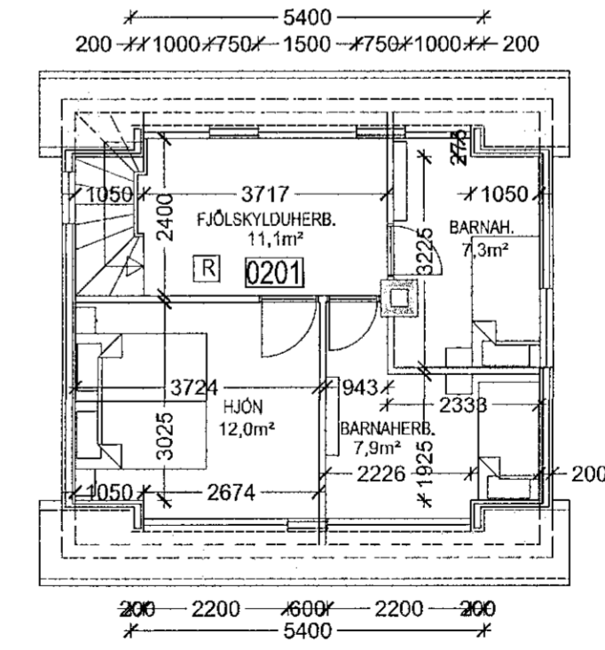
Grunnmynd 1 ris
