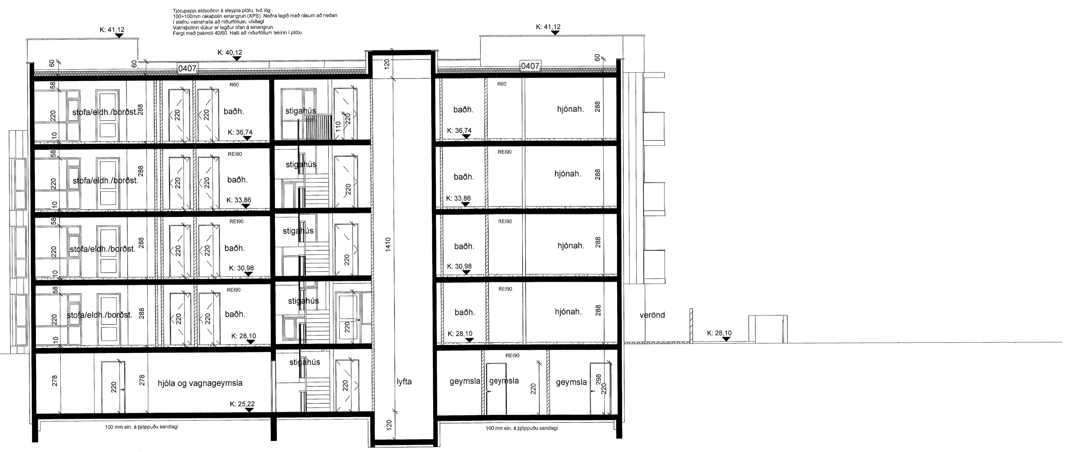
B-B 1 : 100
