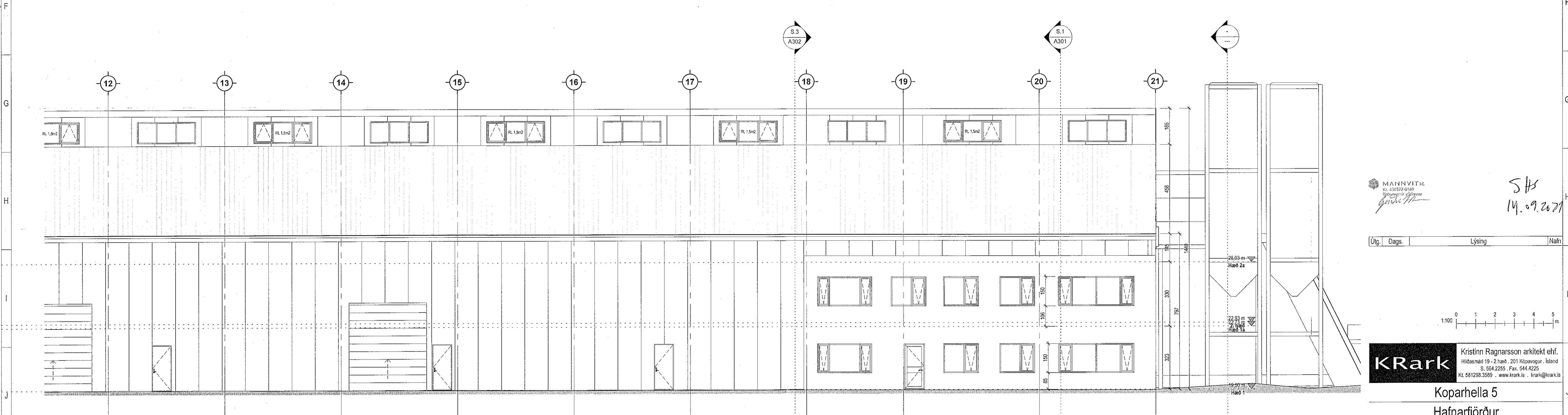
Útlit suður b 1:100
