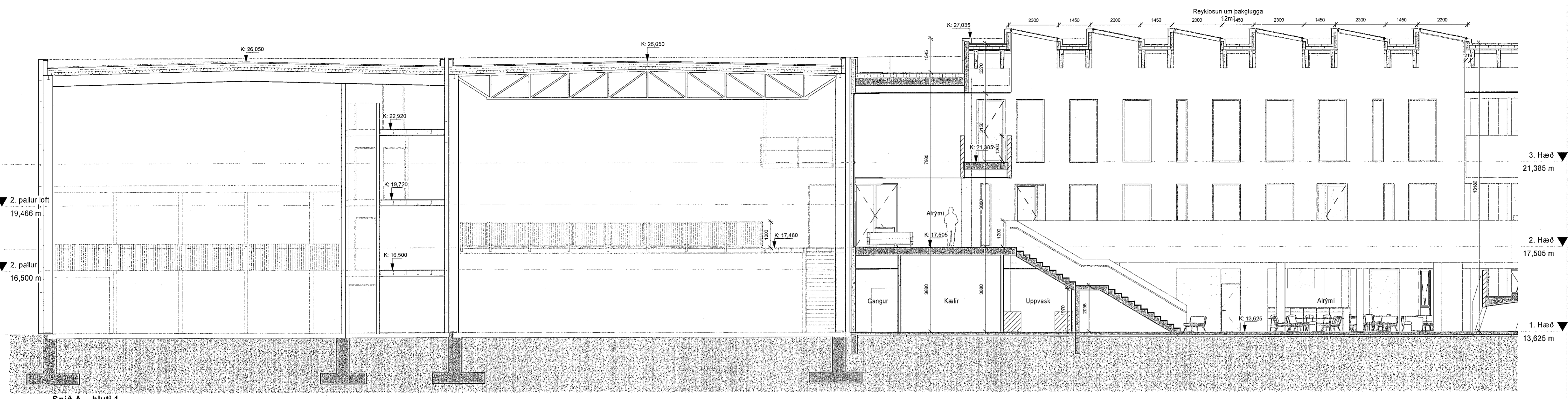
Snið A - hluti 1 1:100
