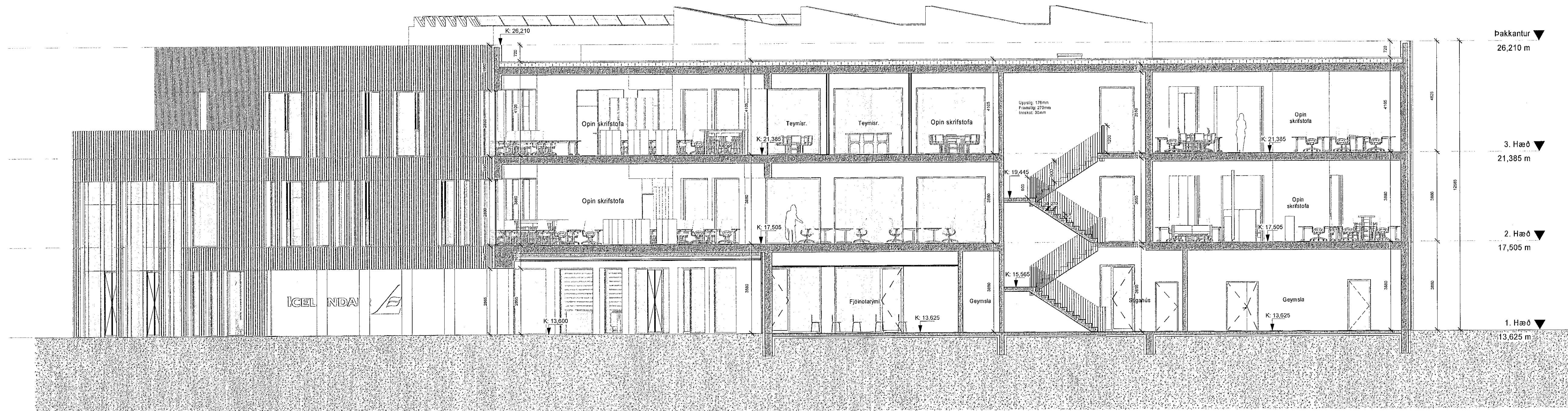
Snið D 1:100
