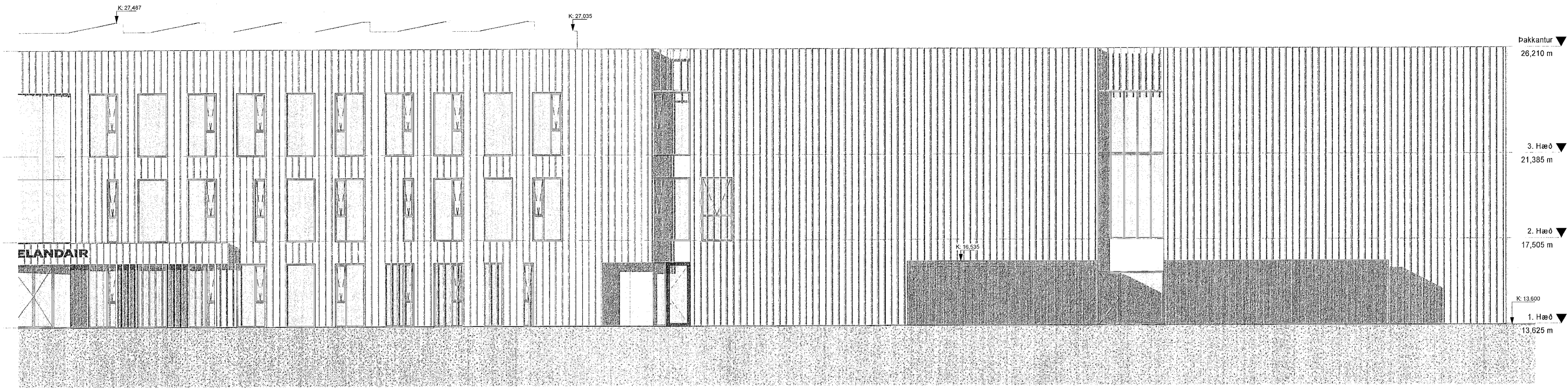
ÚTLIT NORÐUR 1 1:100
