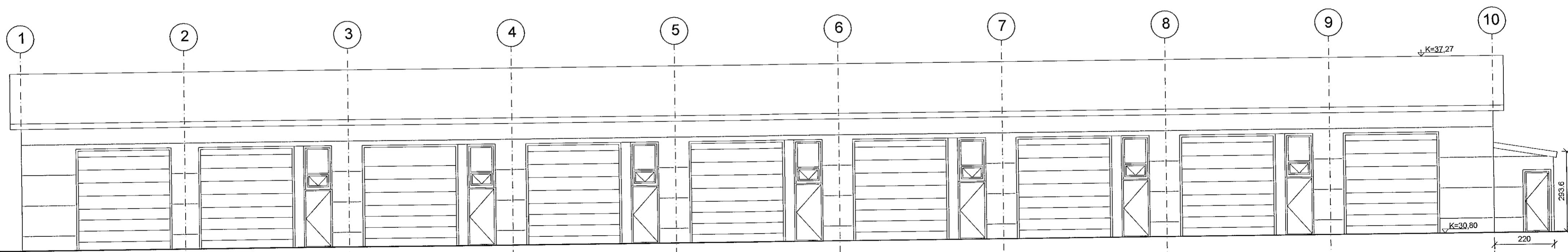
ÚTLIT SUÐUR 1:100
