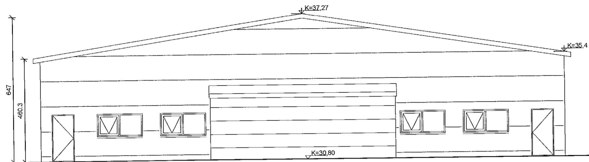
ÚTLIT AUSTUR 1:100
