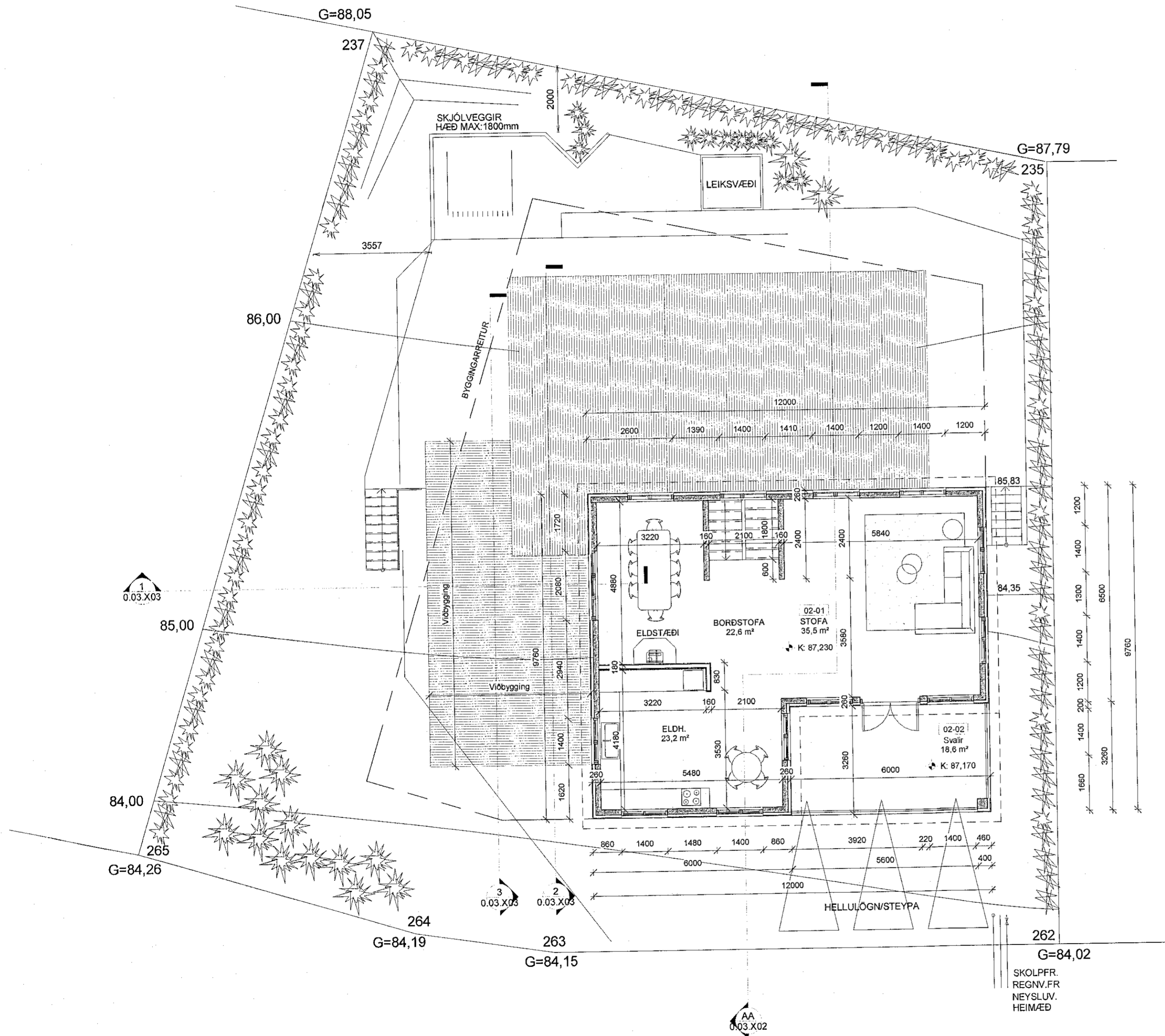
Grunnmynd efri hæð 1:100
