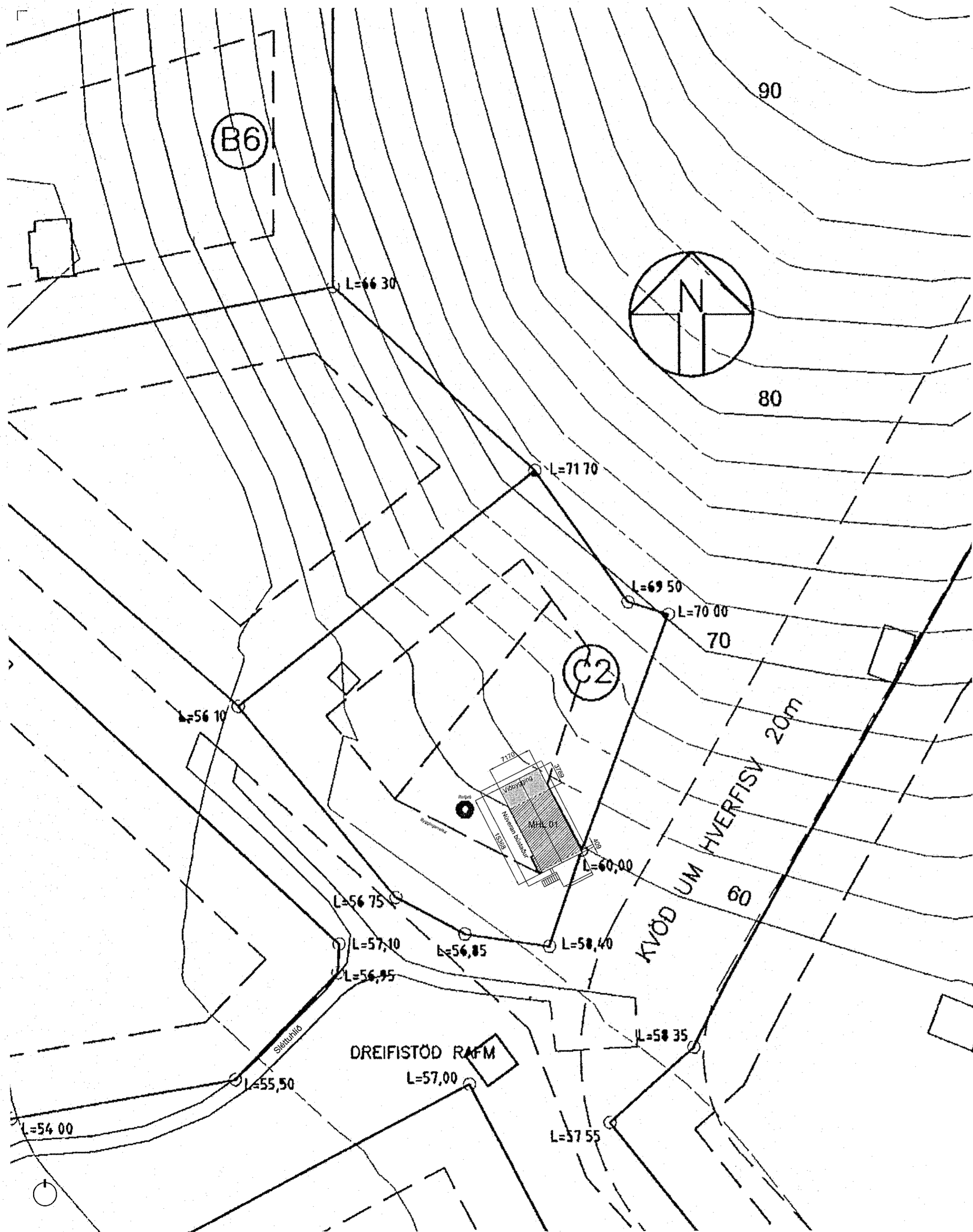
Áfstoðumynd 1:500
