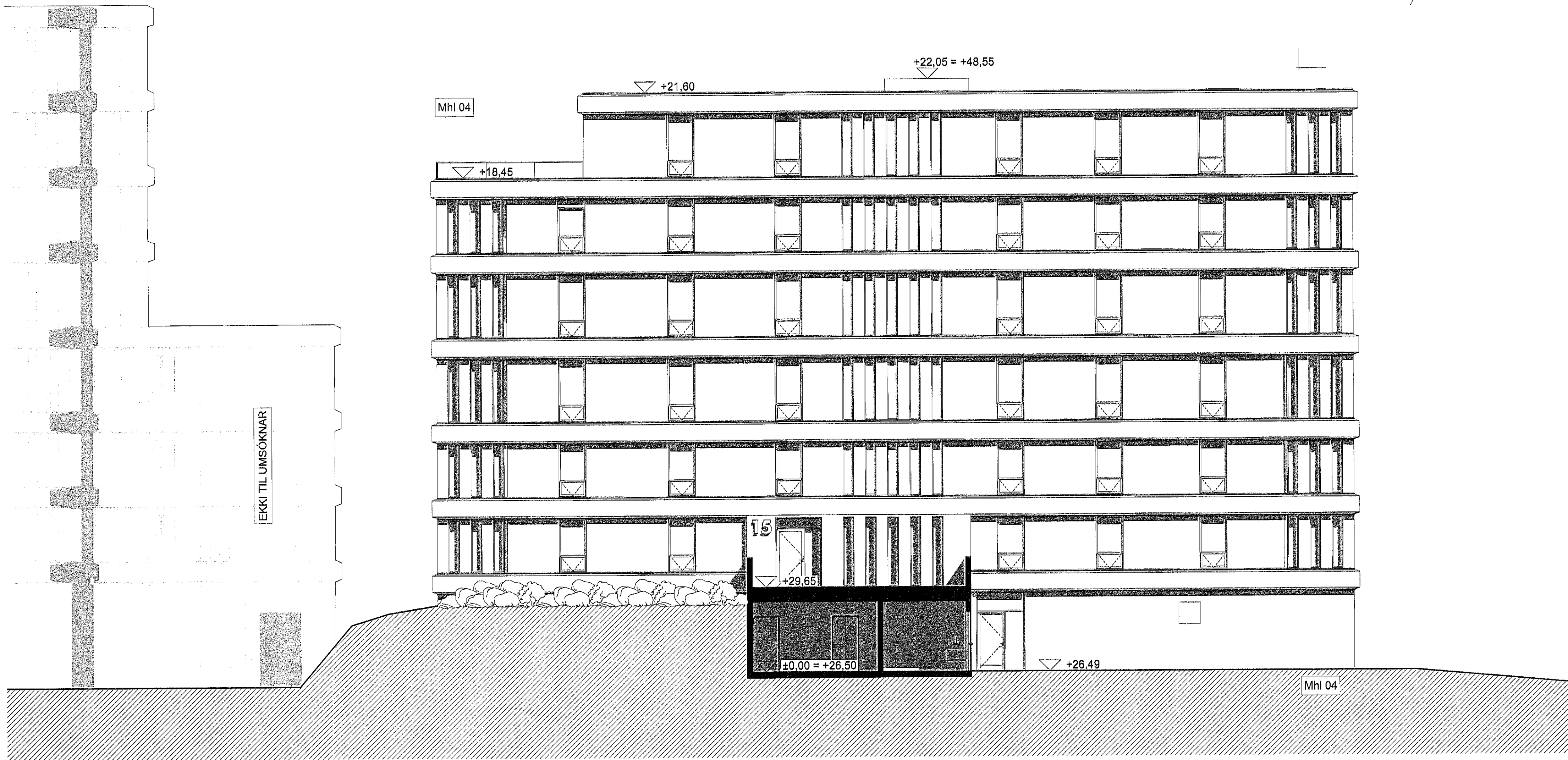
Útlit Norðaustur 1:100
