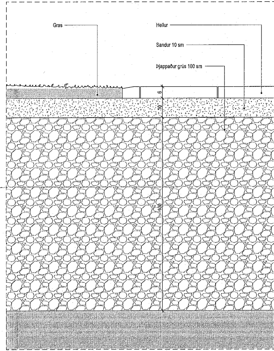
Skýrimynd: uppbygging akumleiða slökkvibíla 1 : 10
