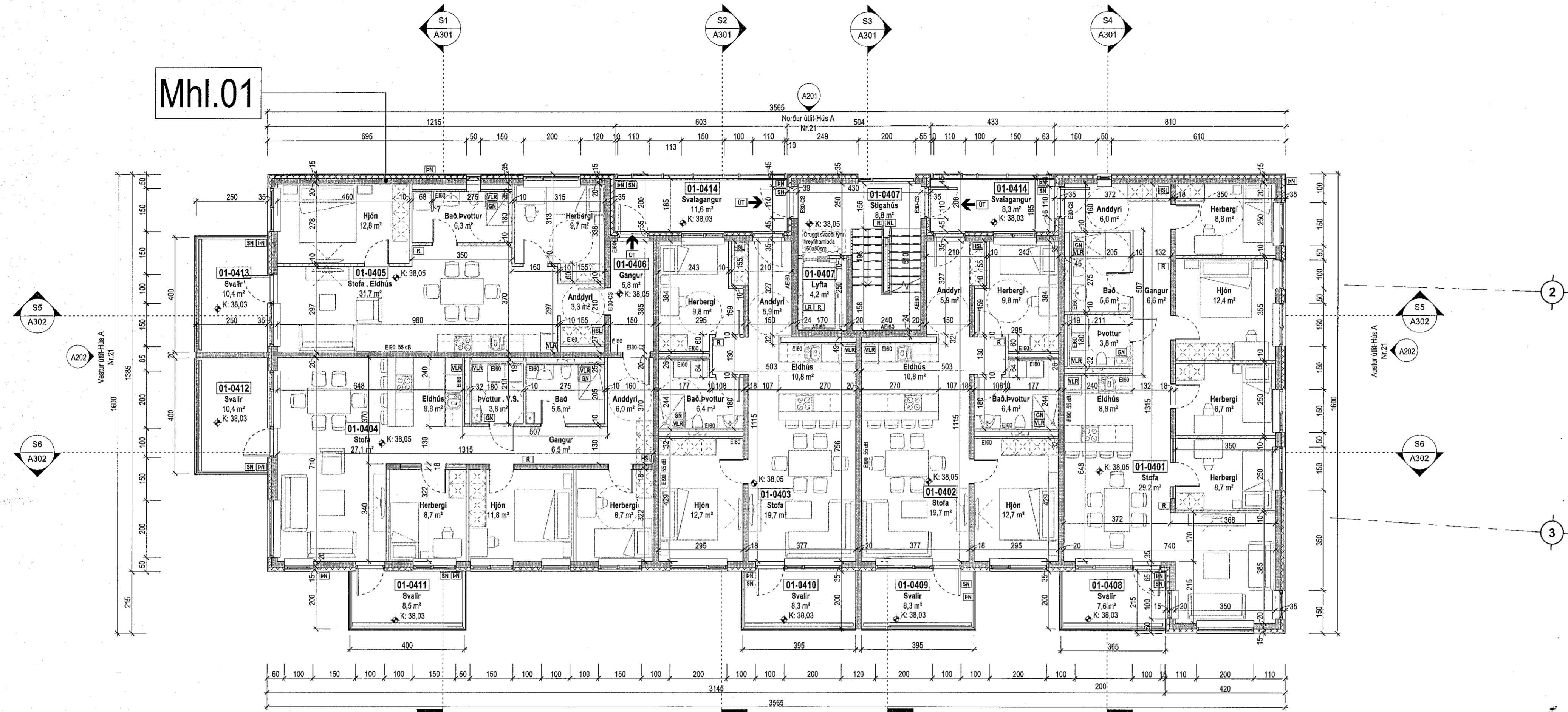
Grunnmynd 4.hæð 1:100
