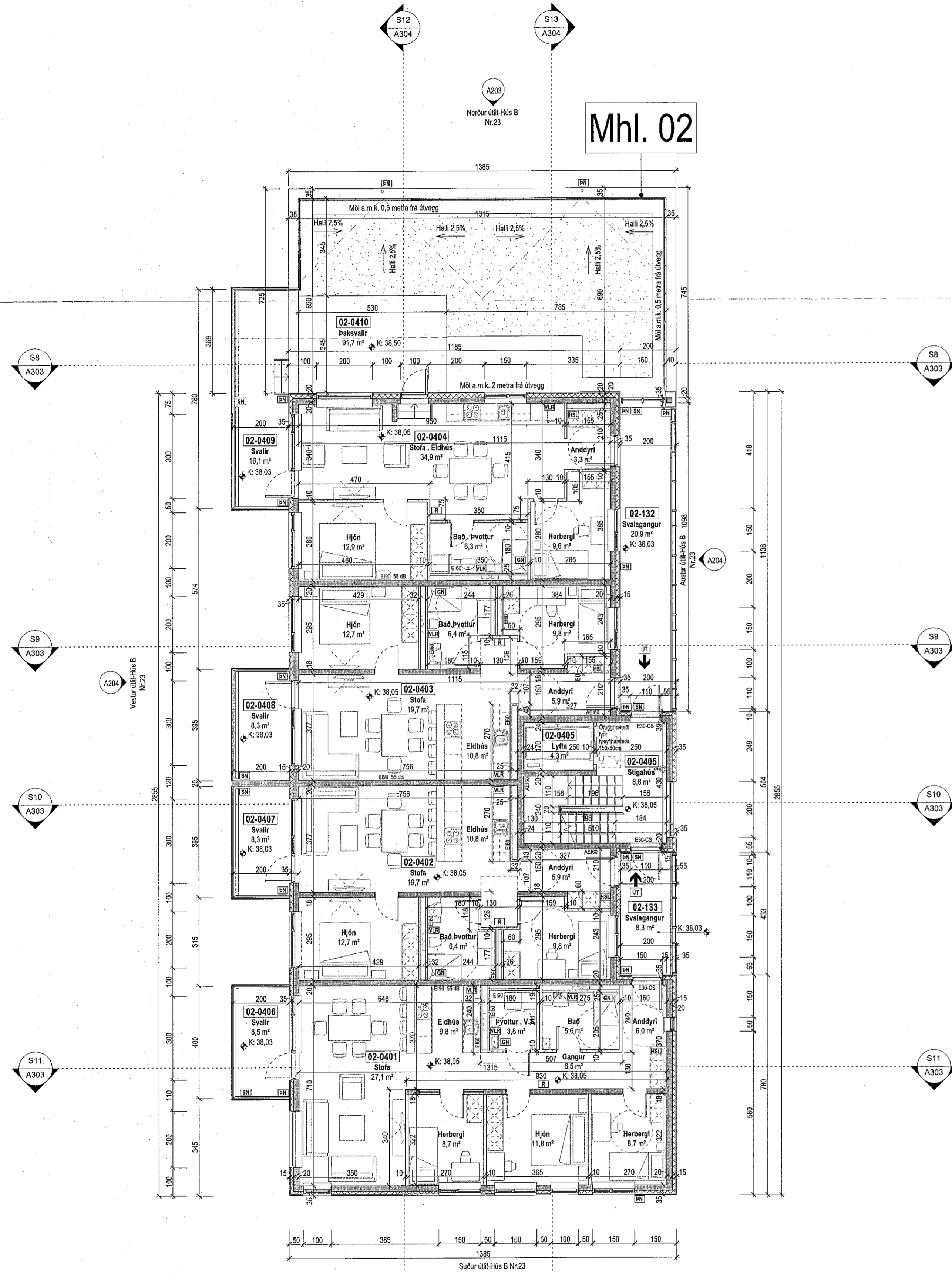
Grunmynd 4.hæð 1:100
