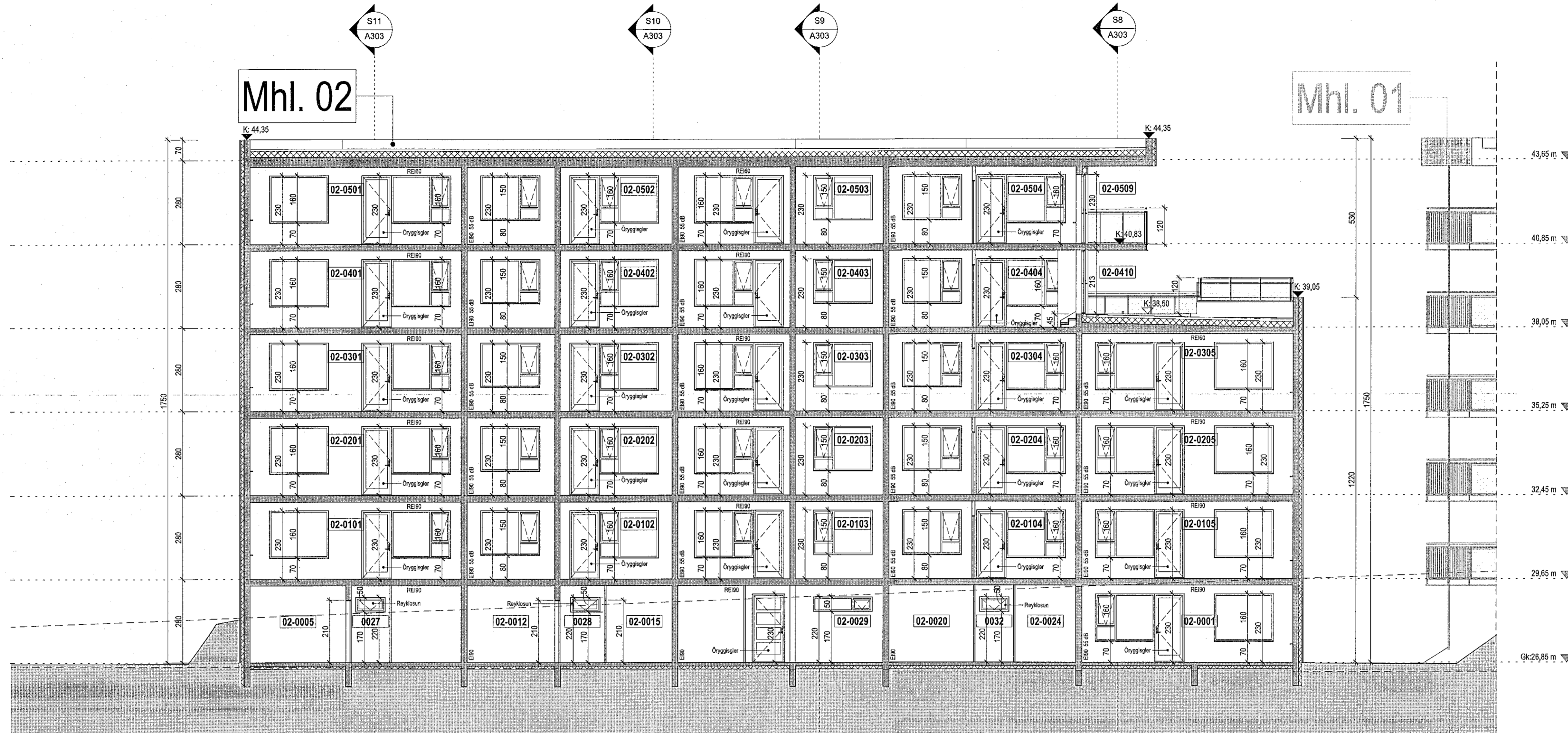
Sníð 12 1:100
