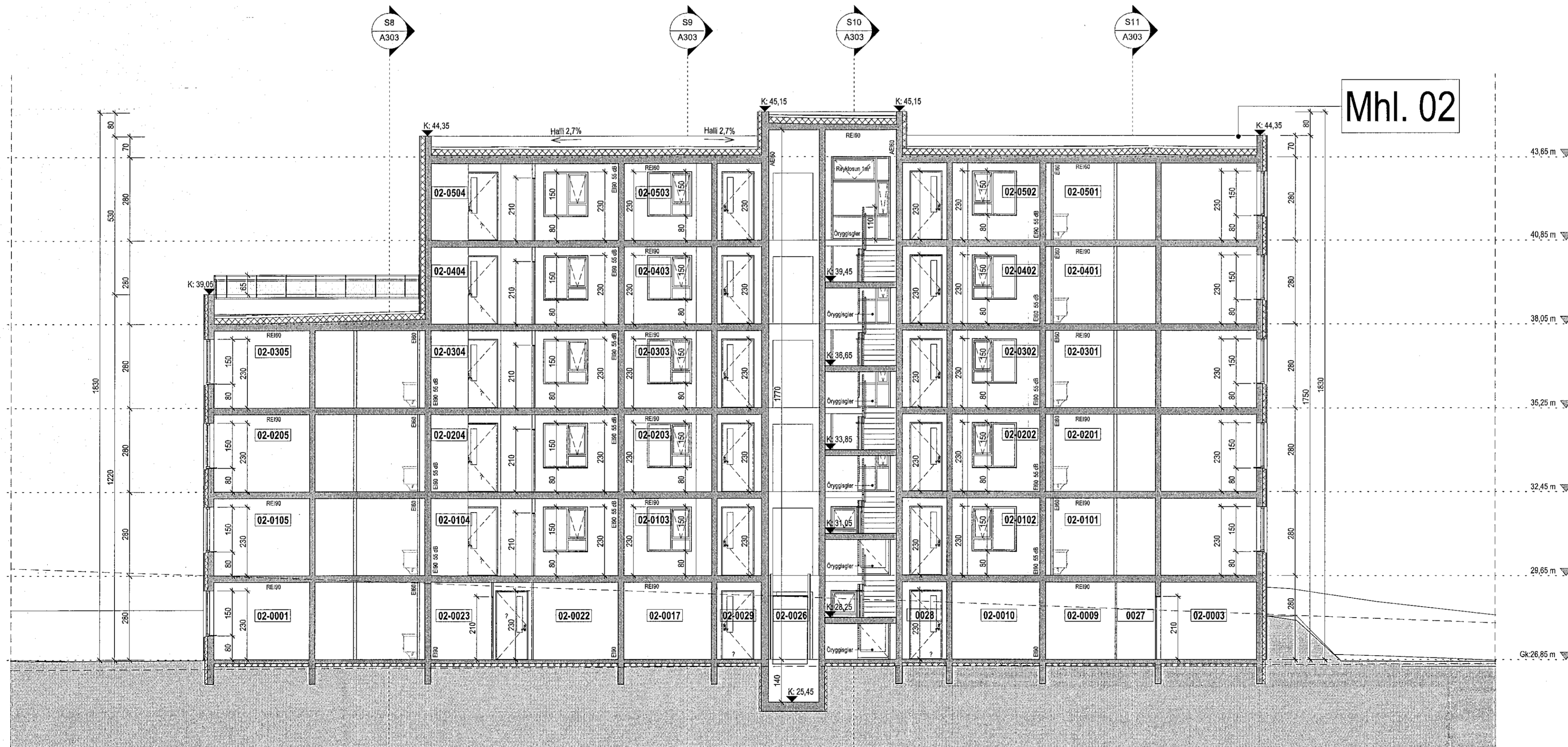
Sníð 13 1:100
