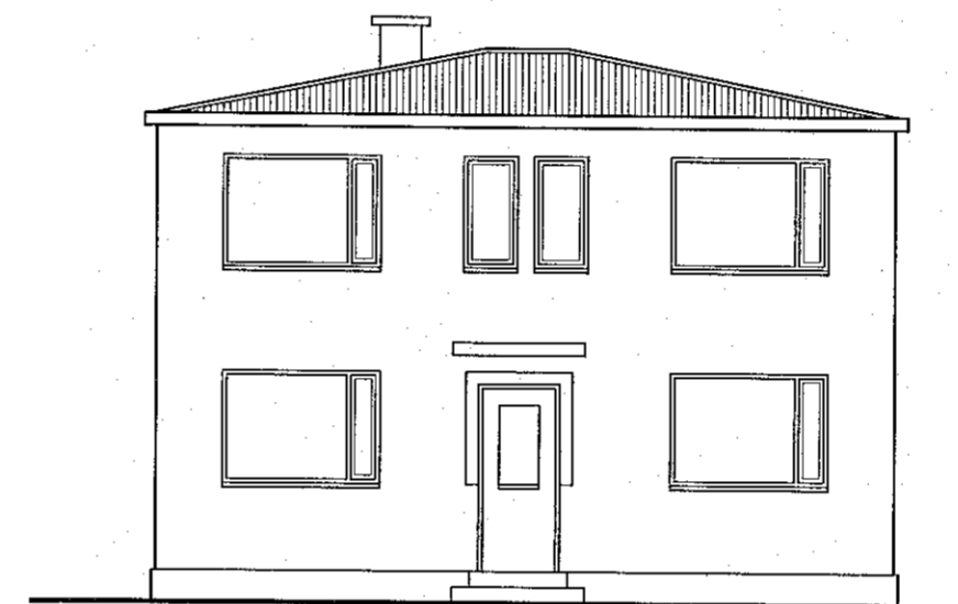
Ásýnd austur mkv. 1:100
