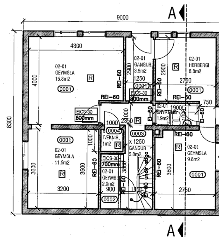
Grunnmynd kjallara mkv. 1:100
