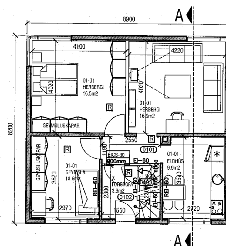
Grunnmynd 1.hæð mkv. 1:100
