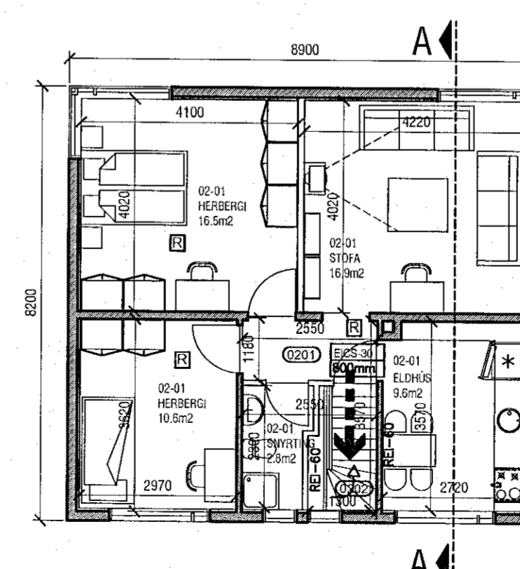
Grunnmynd 2.hæð mkv. 1:100
