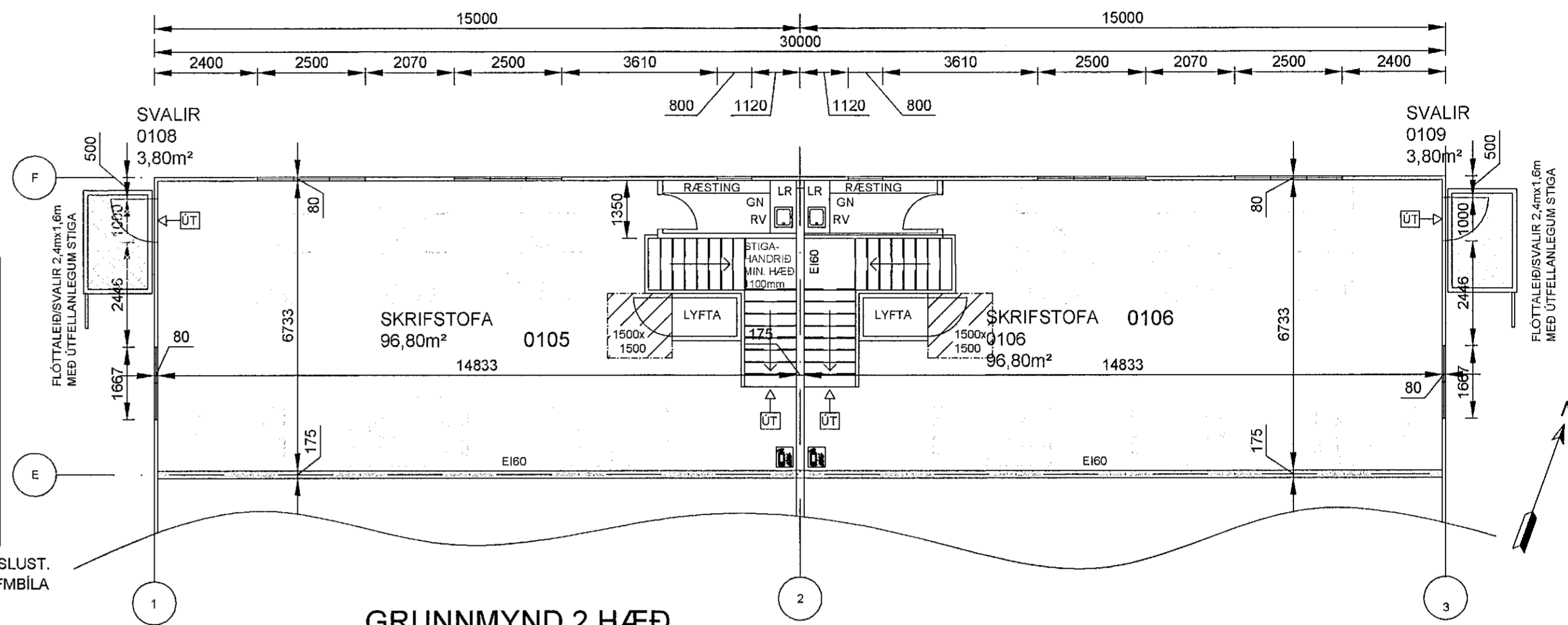
GRUNNMYND 2.HÆÐ 1:100 (A1)
