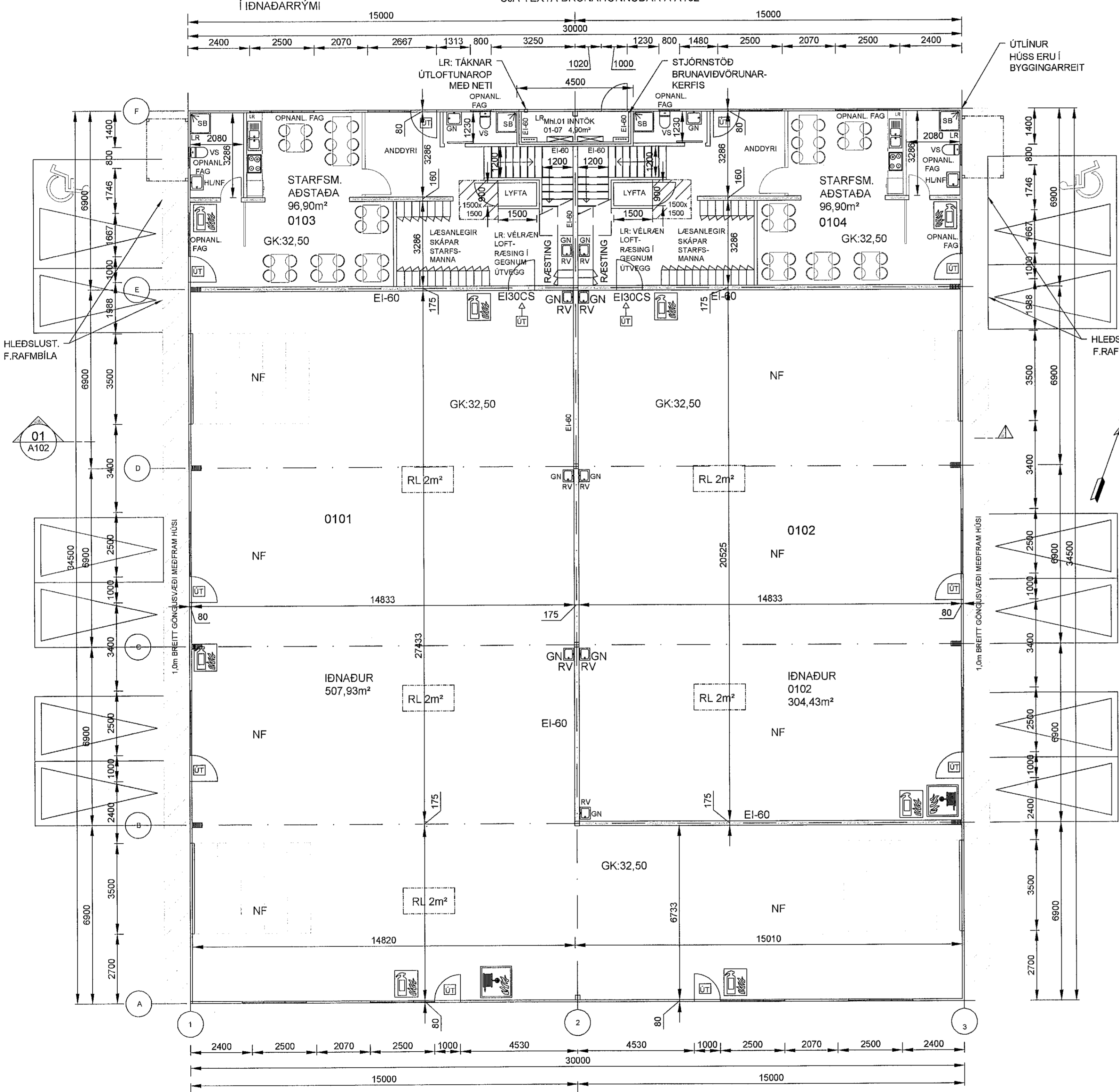
GRUNNMYND 1.HÆÐ 1:100 (A1)
