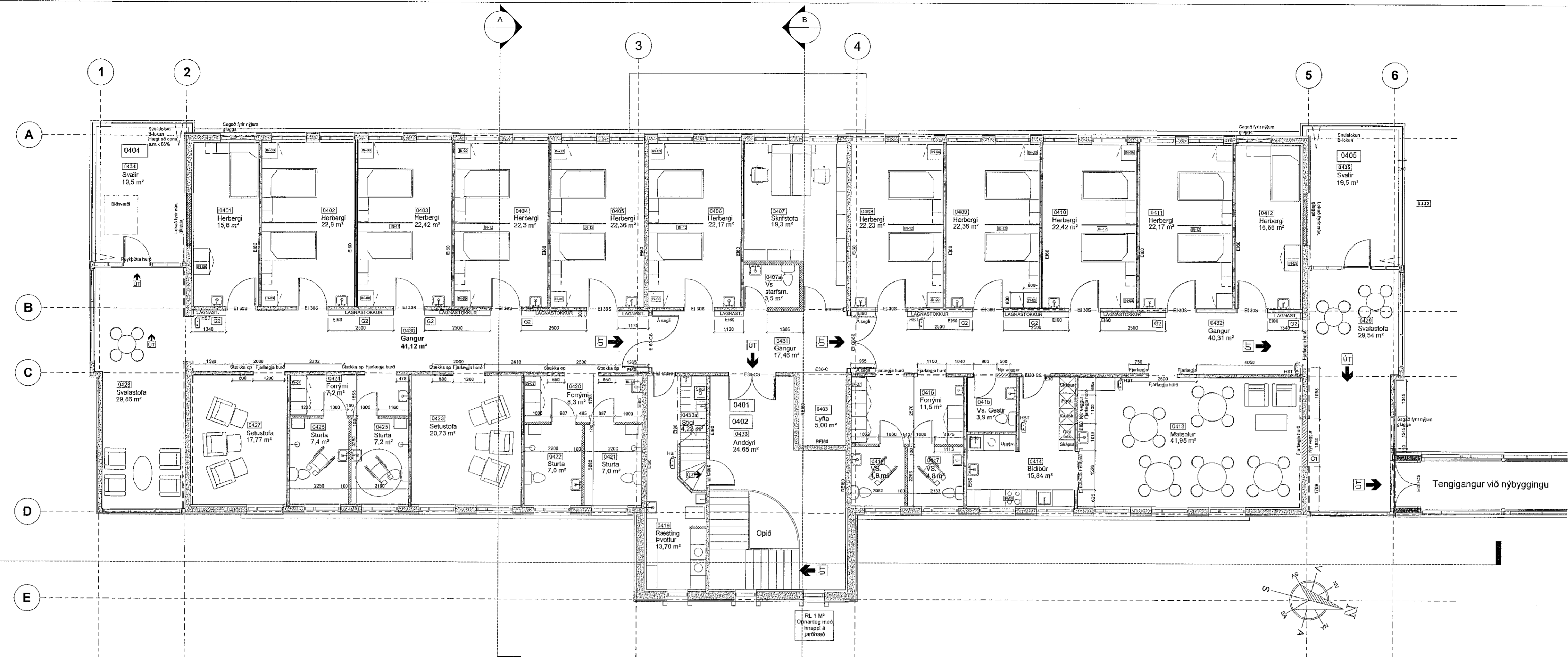
GRUNNMYND 4. HÆÐAR
