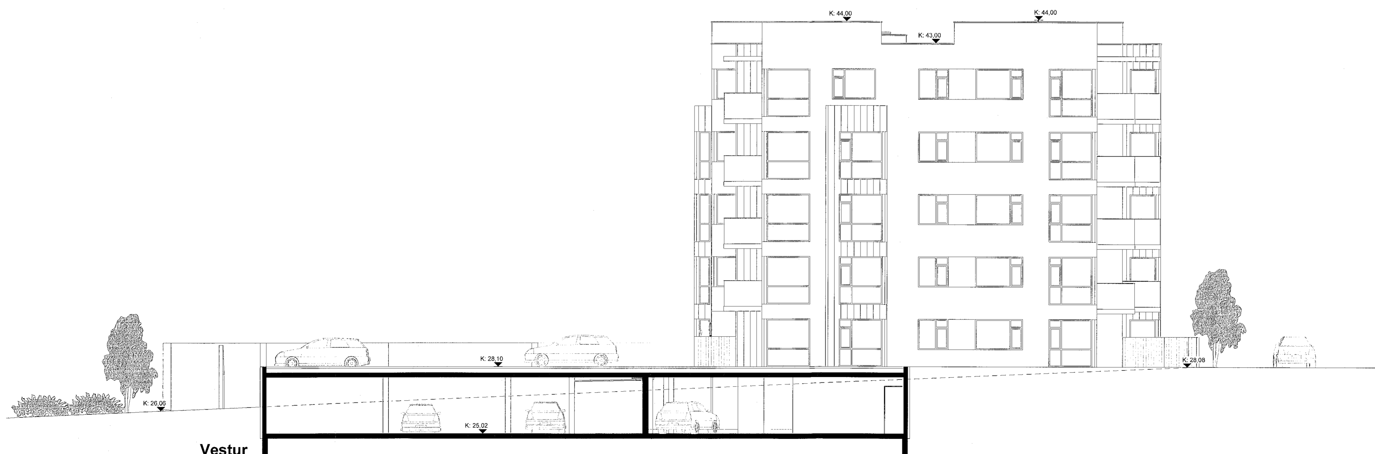
Vestur 1 : 100
