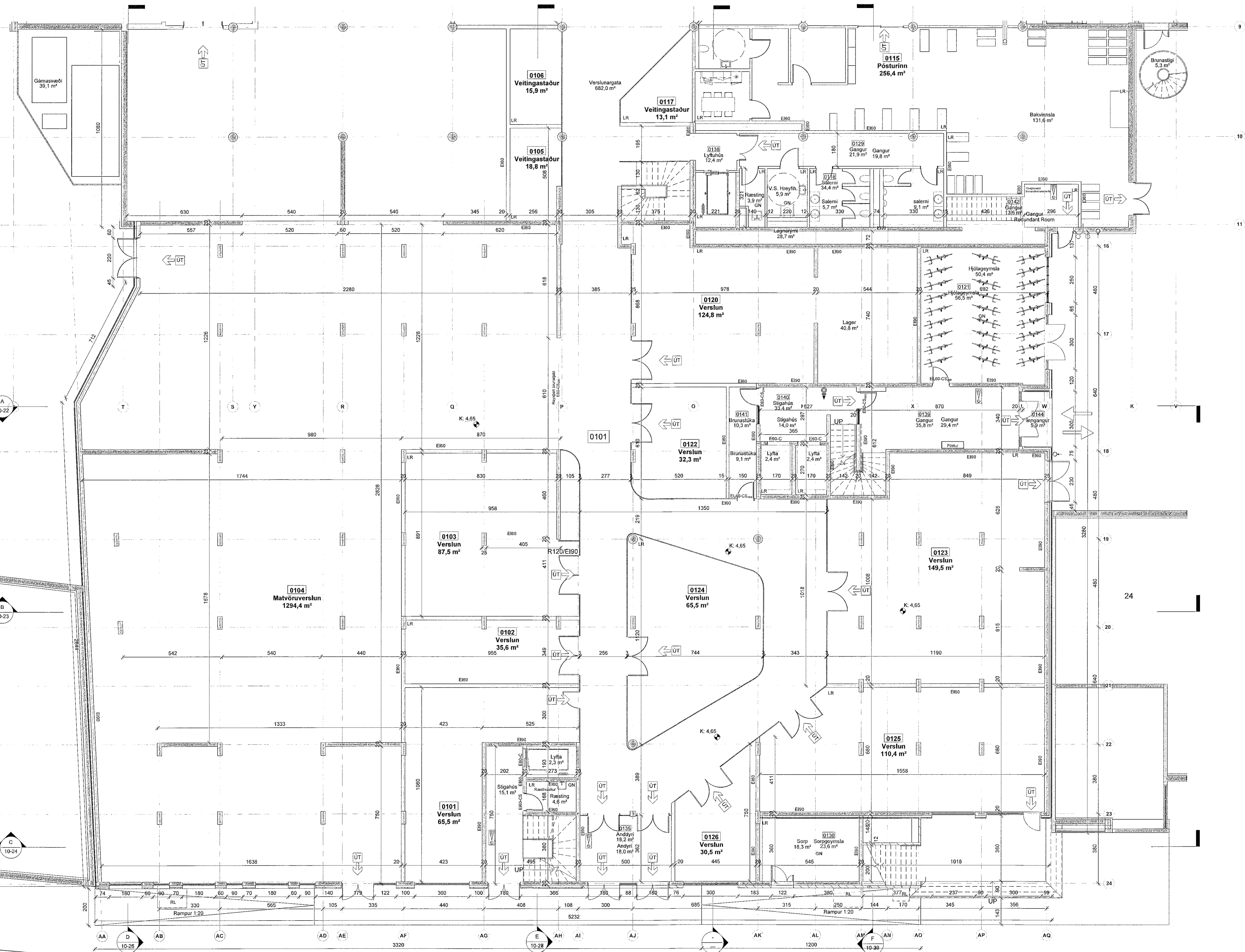
Grunnmynd 1. hæð - Nýbygging 1 : 100
