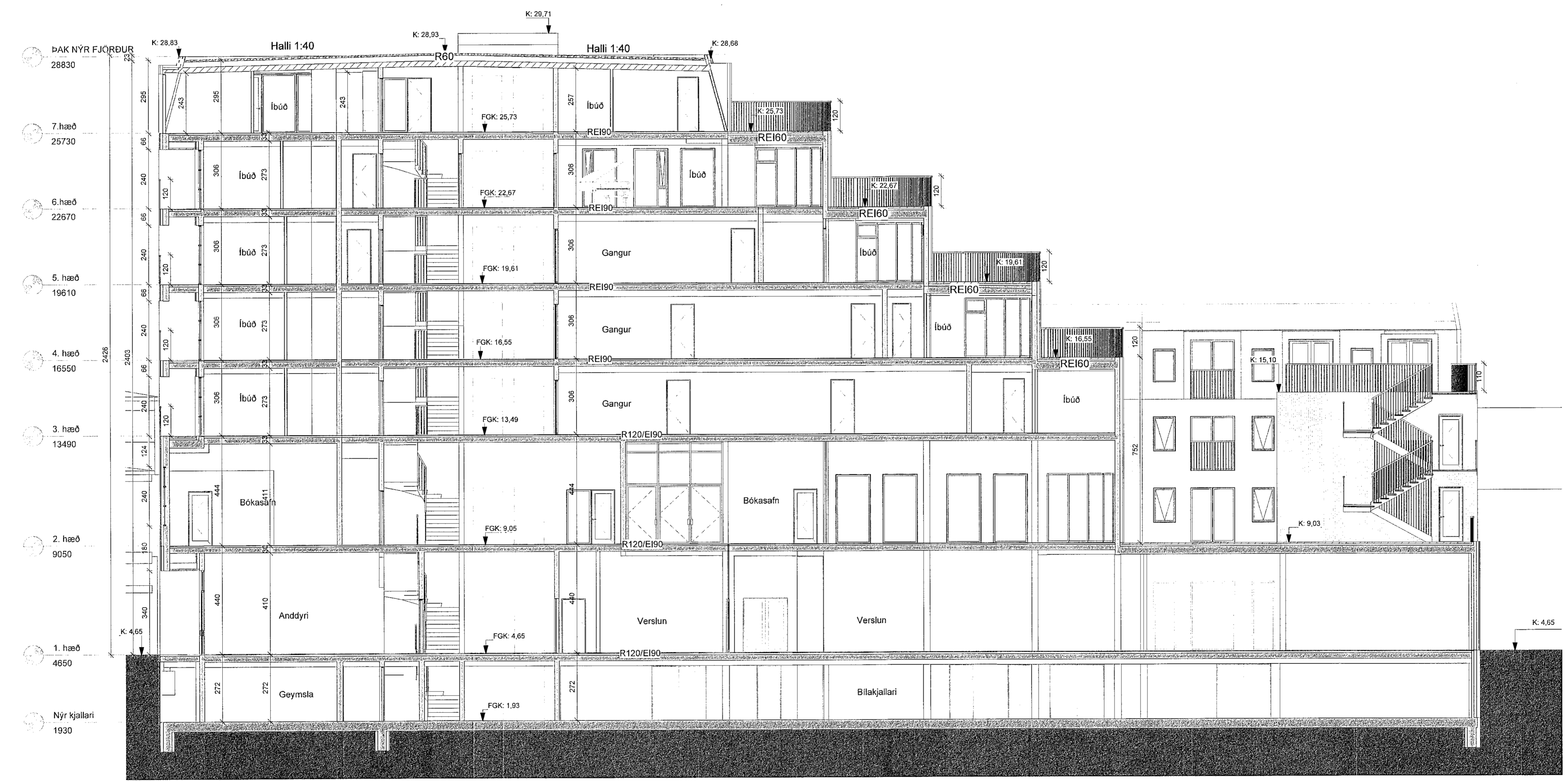
Sneiðing A-A 1:100 1:100
