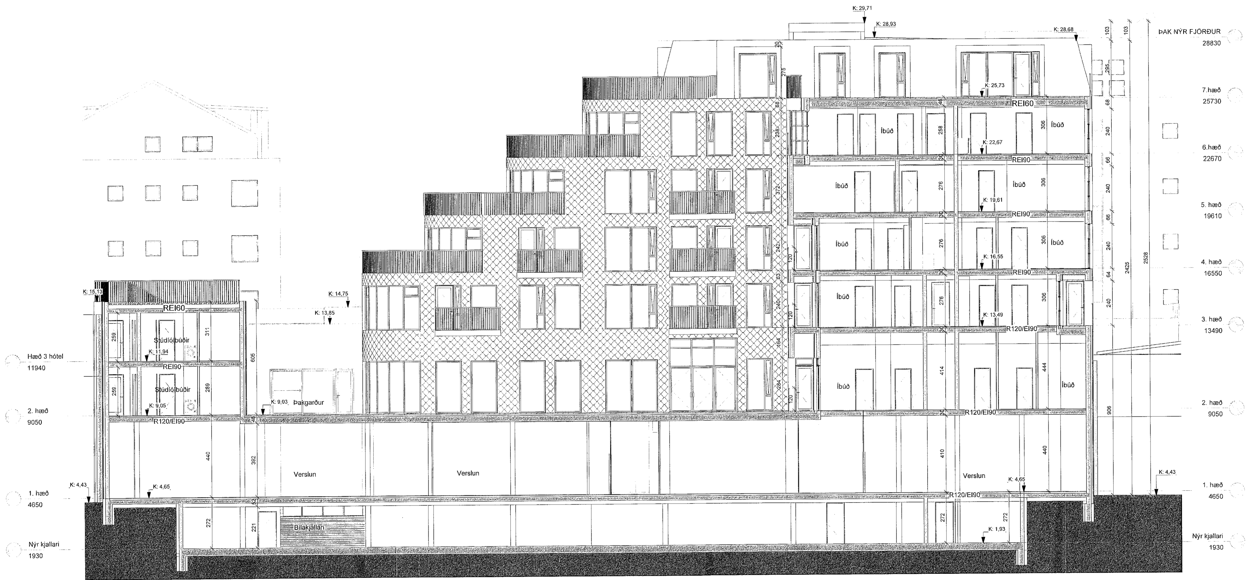
Sneiðing B-B 1:100
