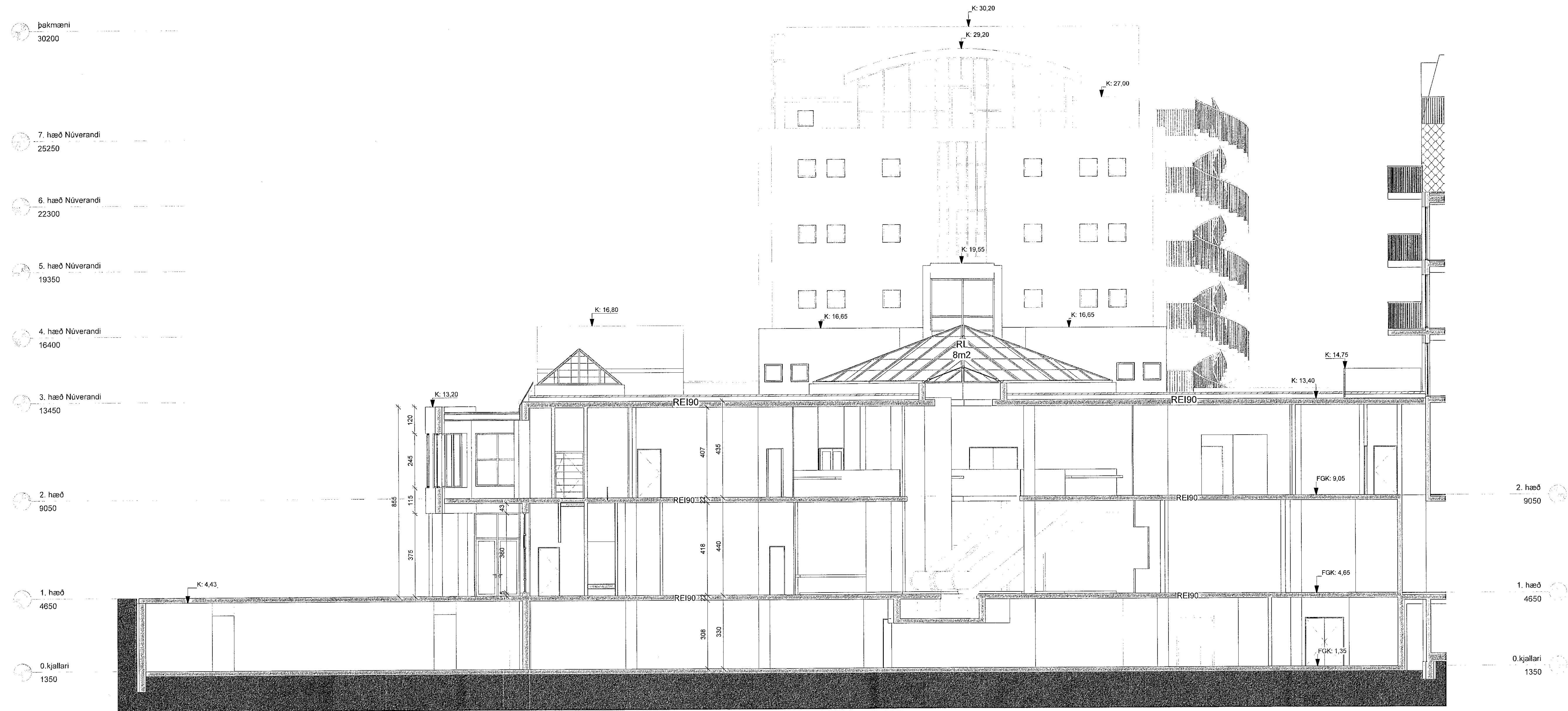
Sneiðing E-E 1 : 100
