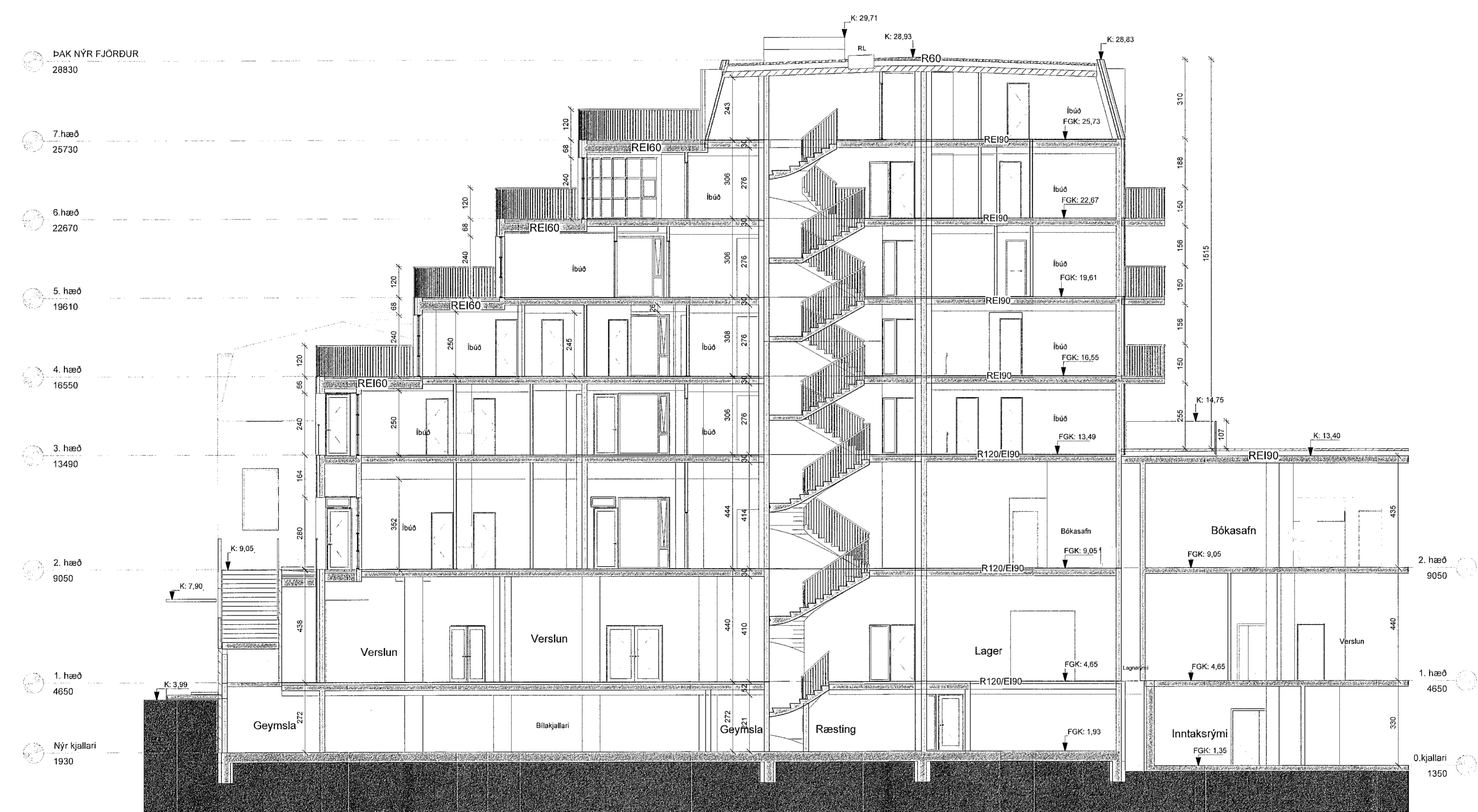
Sneiðing F-F Nýbygging 1: 100
