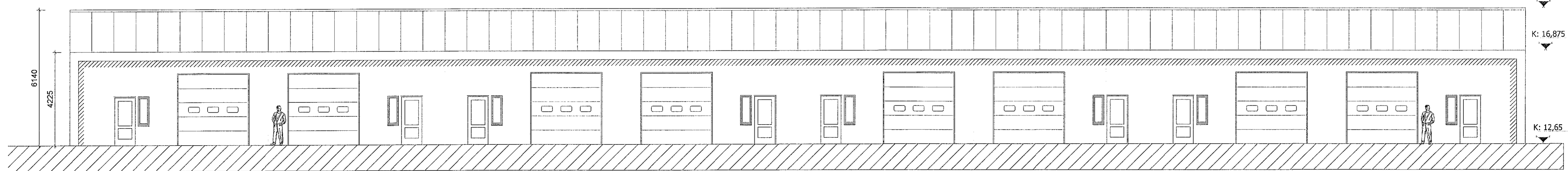
ÚTLIT AUSTUR 1:100
