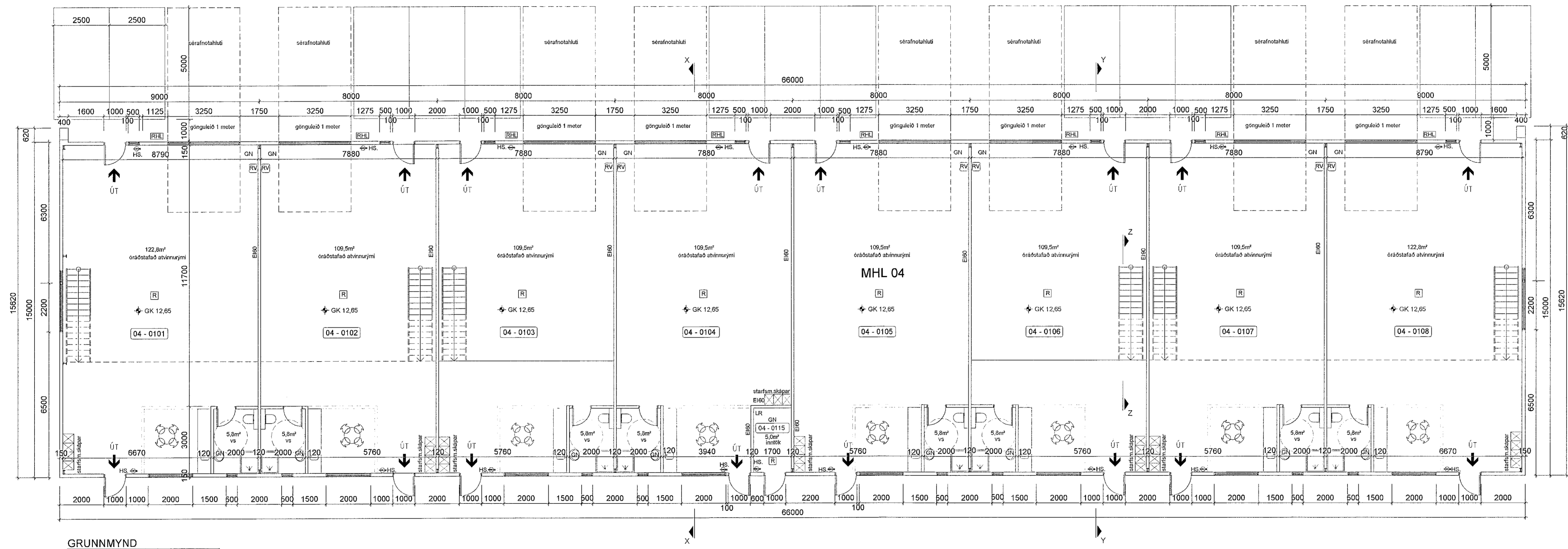
GRUNNMYND 1:100
