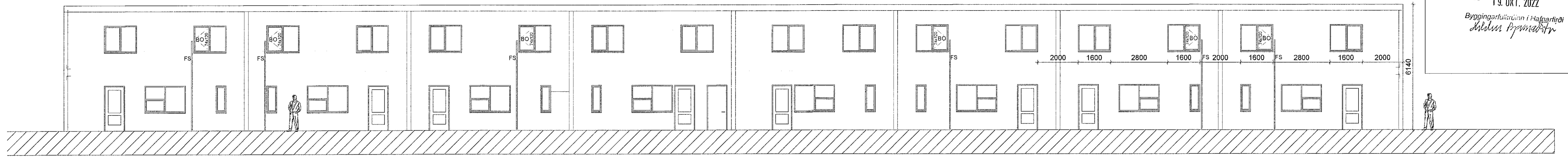
ÚTLIT VESTUR 1:100
