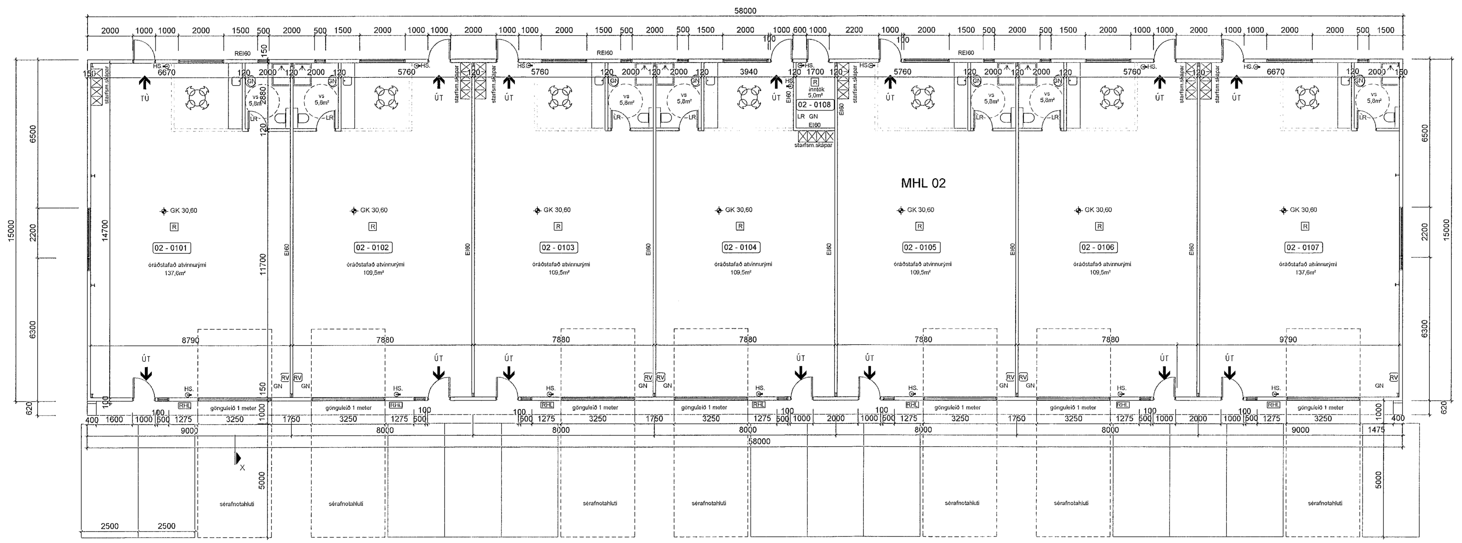
GRUNNMYND 1:100
