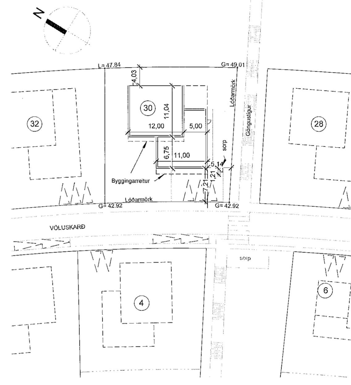
Afstöðumynd 1:500
