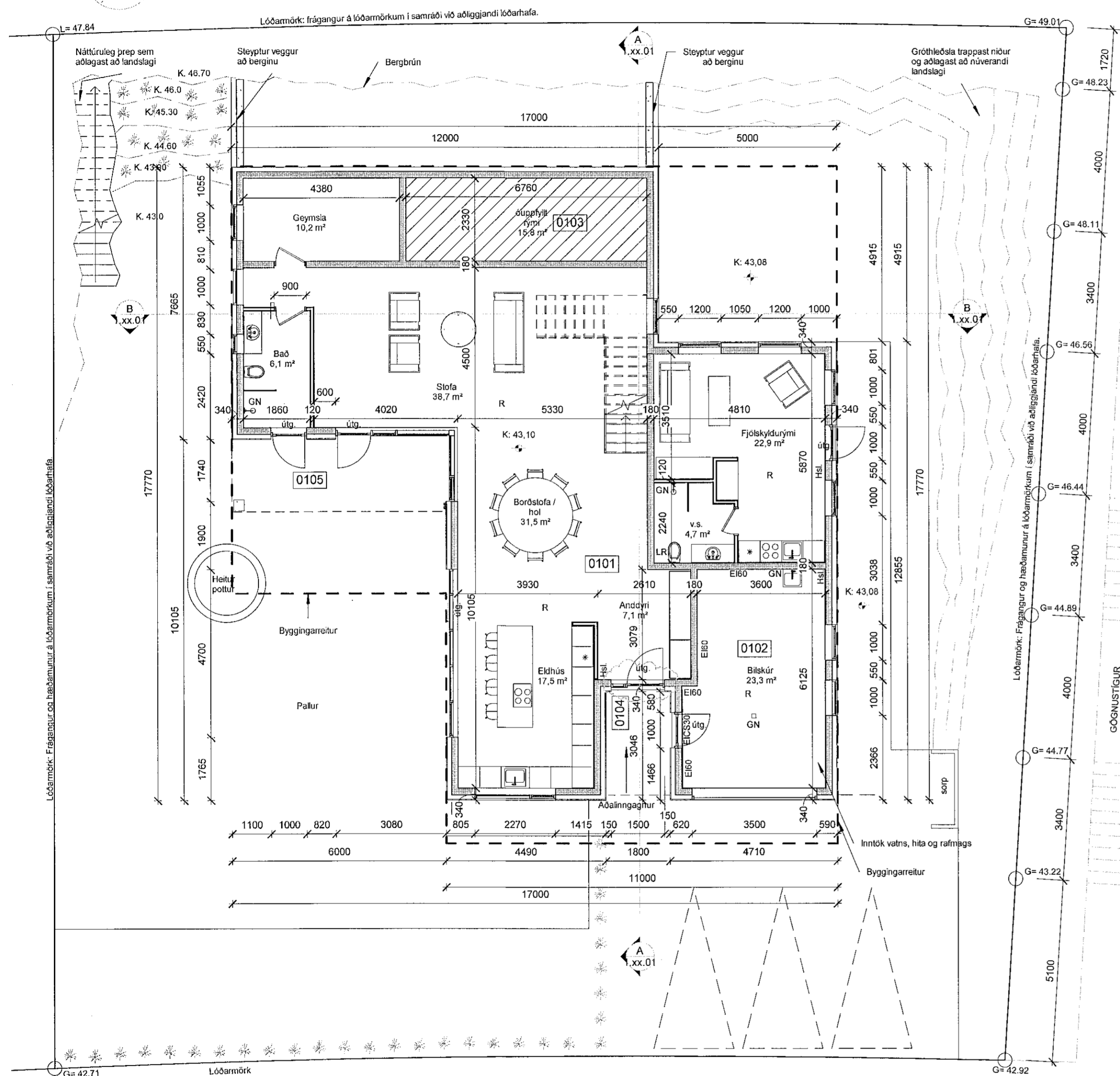
Afstöðumynd 1:500
