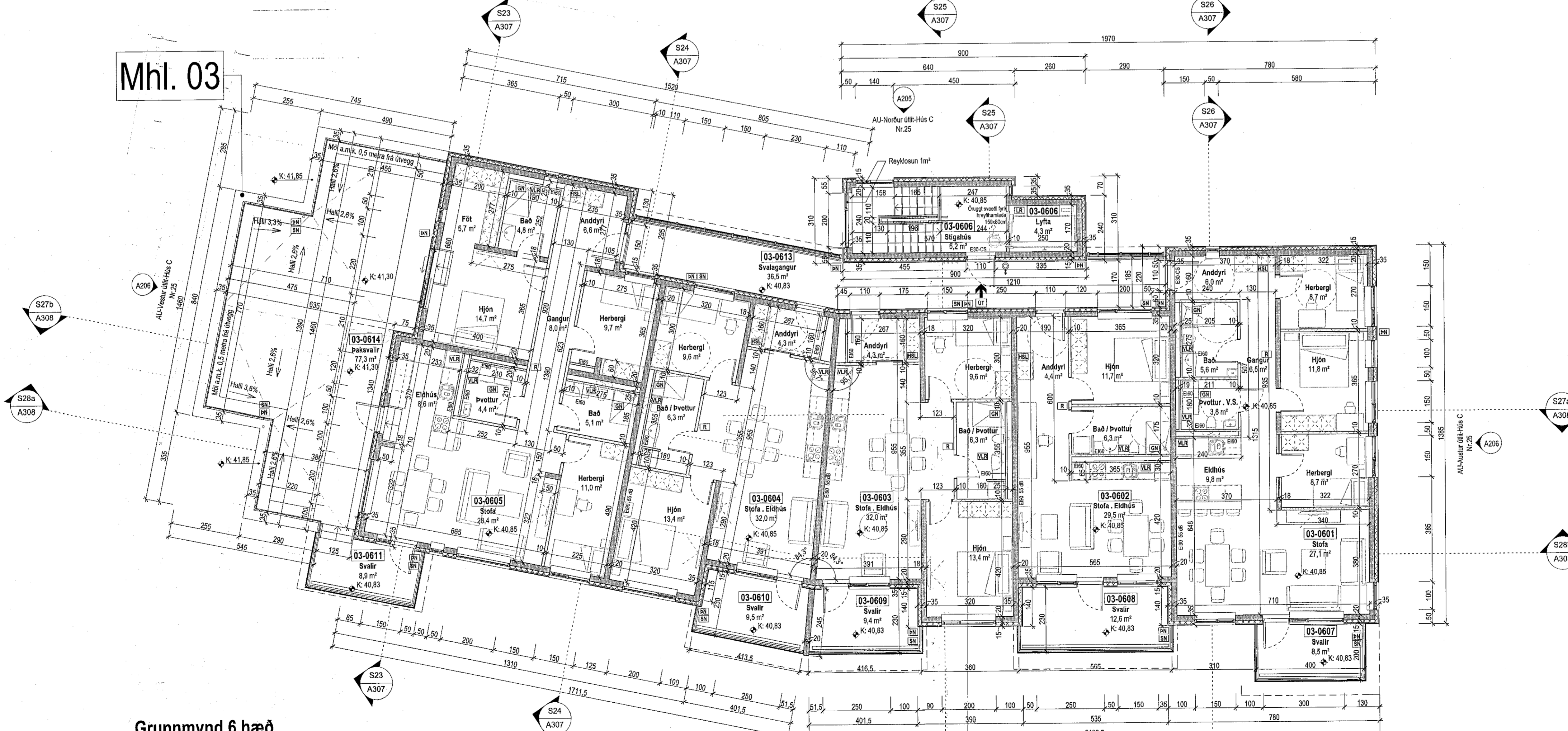
Grunnmynd 6. hæð 1:100
