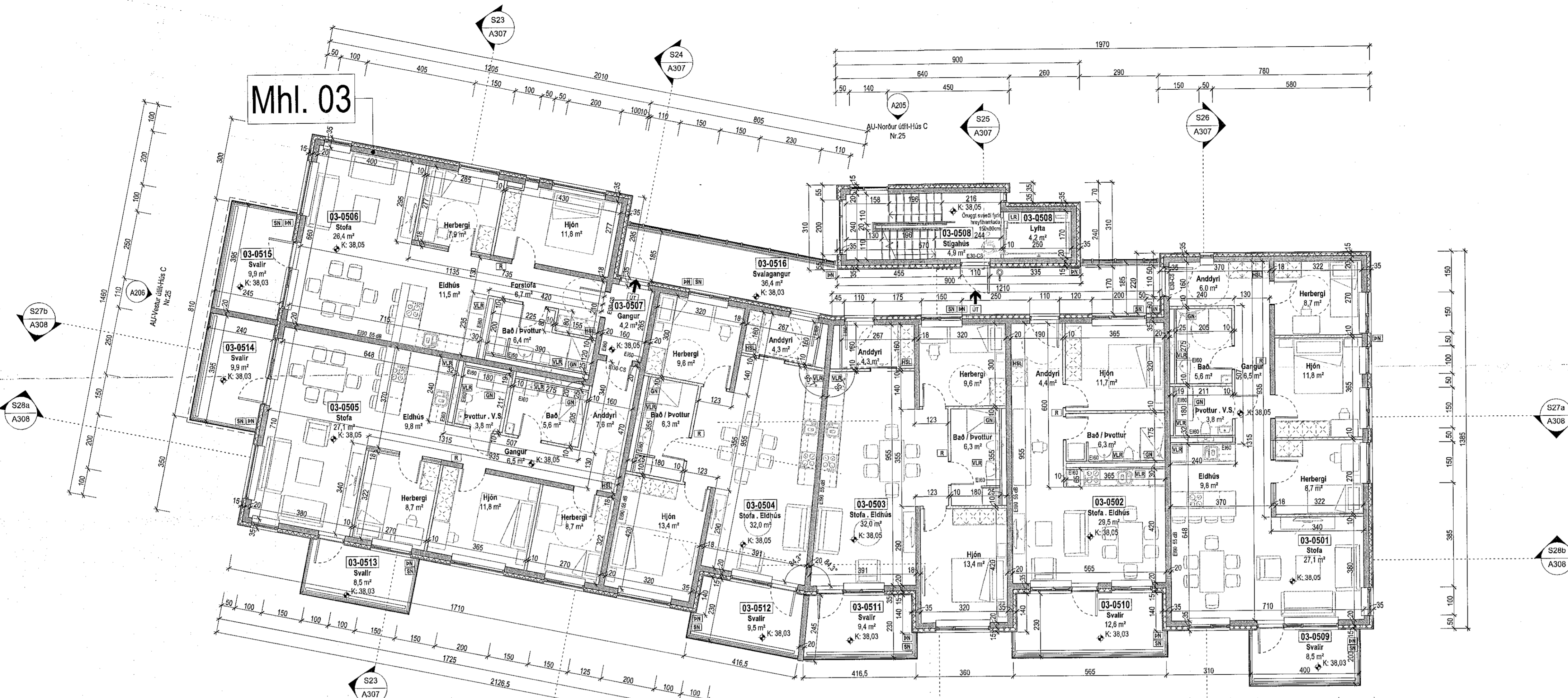
Grunnmynd 5. hæð 1:100
