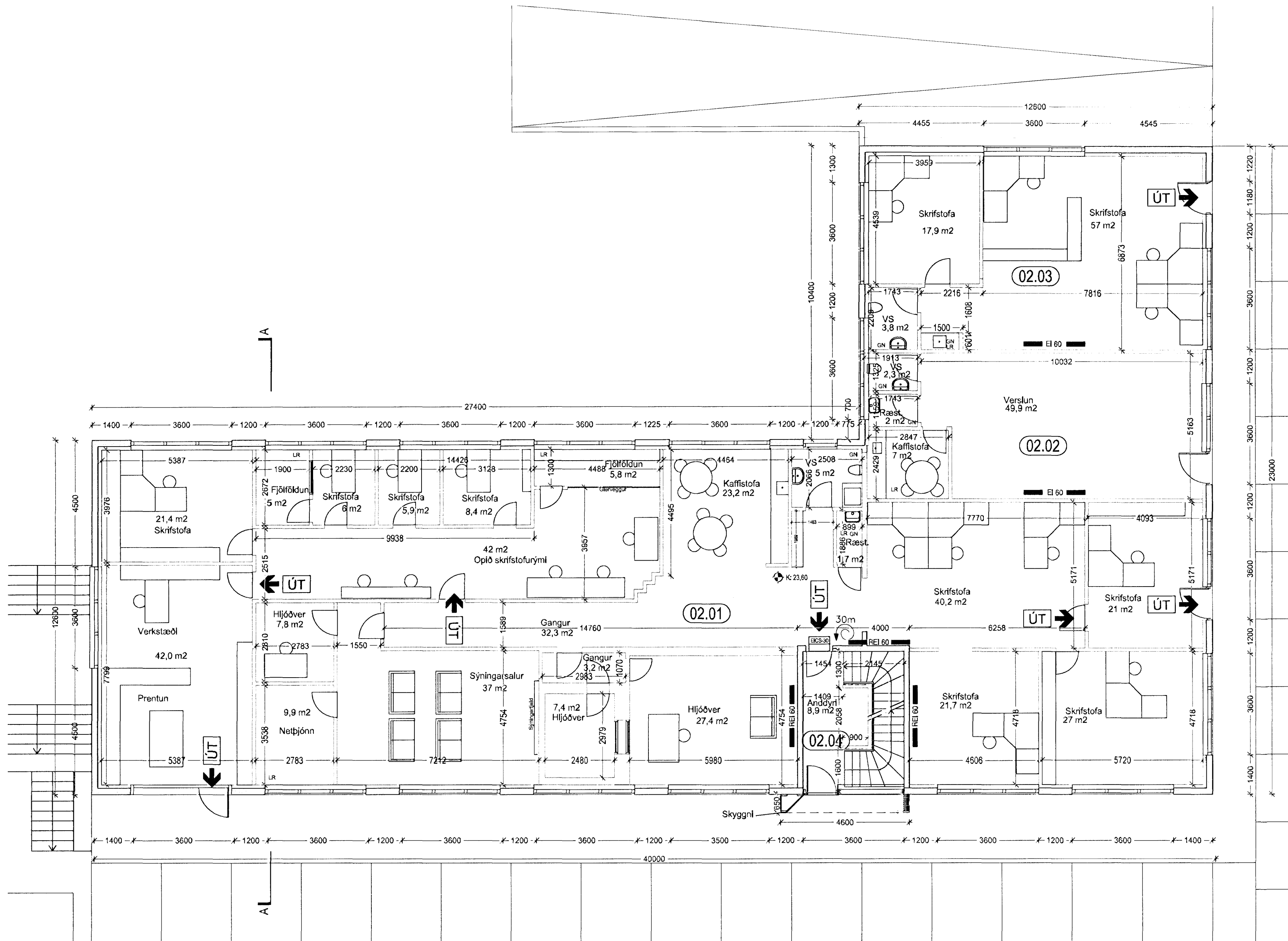
GRUNNMYND 2. HÆÐAR MKV 1:100
