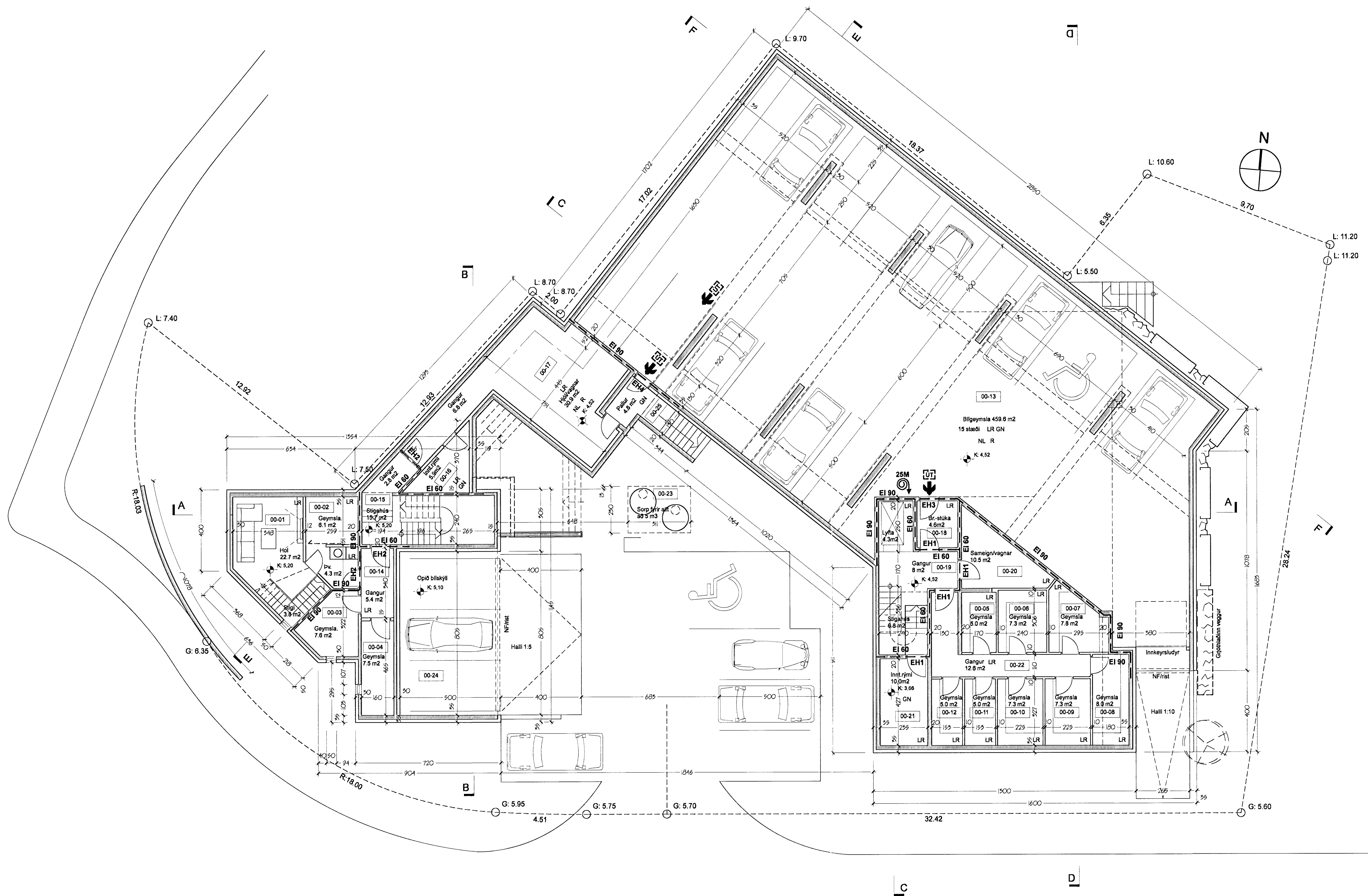
Grunnmynd kjallara mkv.1:100
