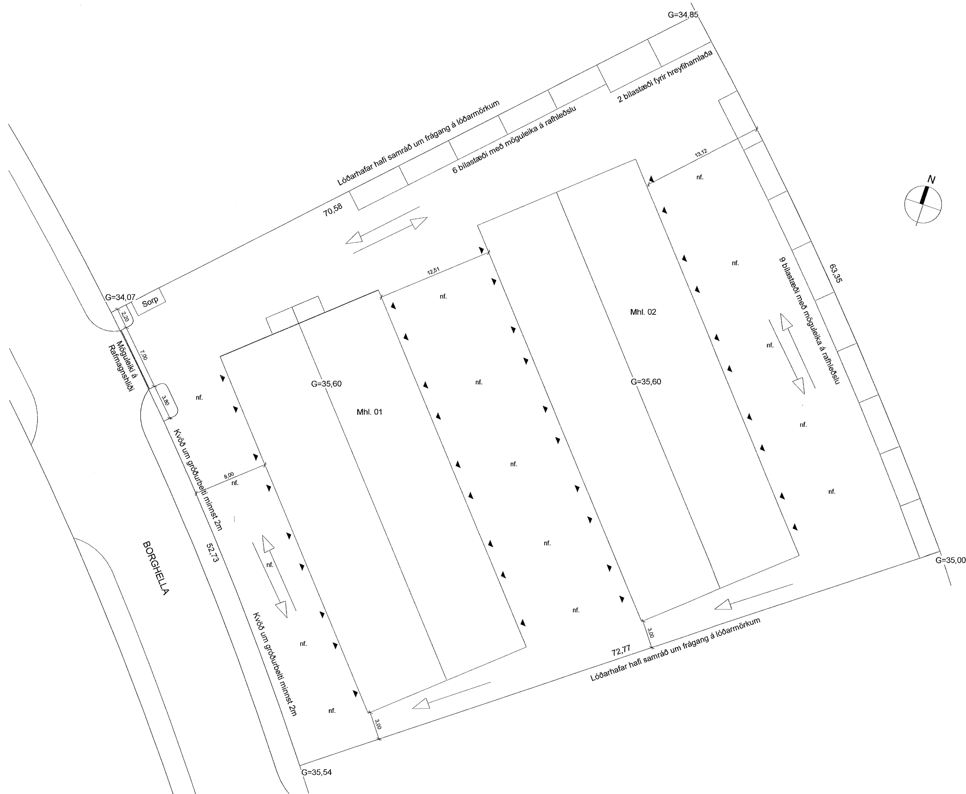
1 Lóðarmynd 1 : 200
