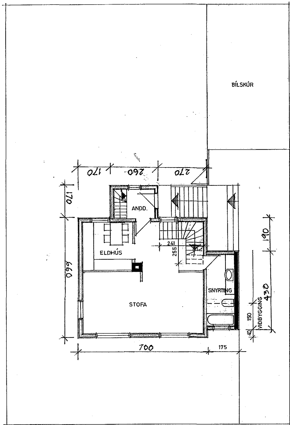
GRUNNMYND AÐALHÆÐAR 1:100
