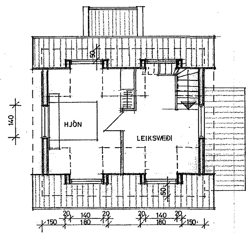
GRUNNMYND RISHÆÐAR 1:100
