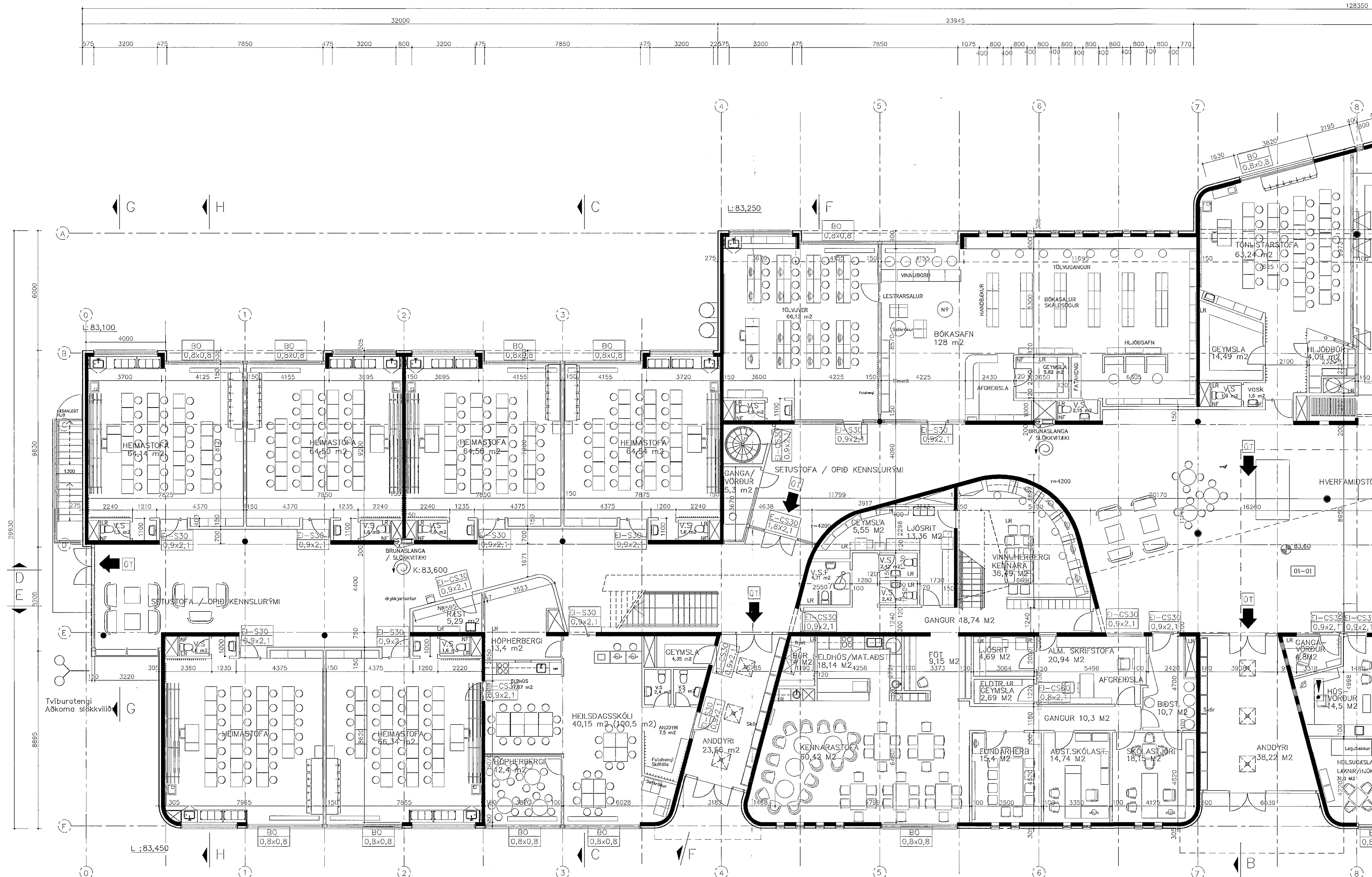
GRUNNMYND 1.HÆÐ MKV. 1:100
