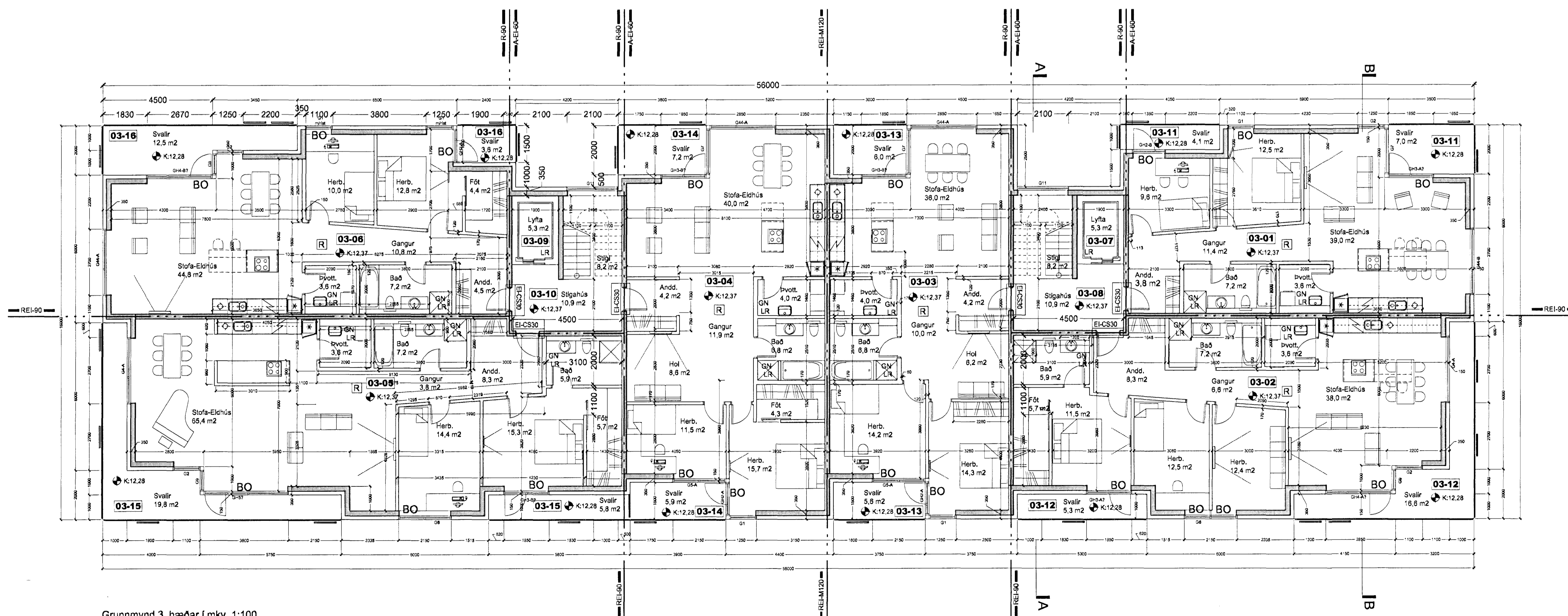
Grunnmynd 3. hæðar í mkv. 1:100
